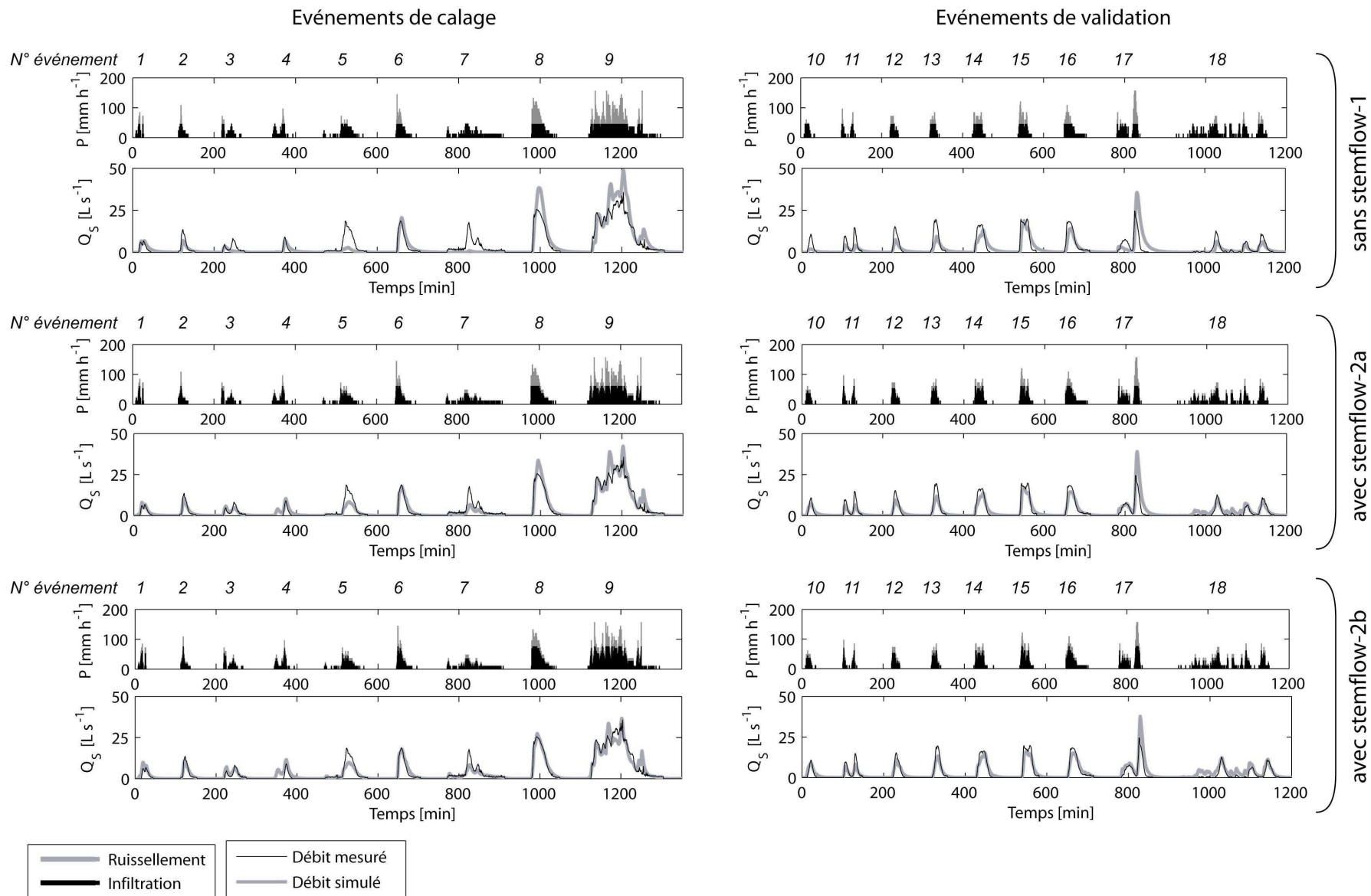
Figure 6-7 Résultats des simulations pour le calage et la validation ; les différents événements sont représentés sur le même axe de temps.
