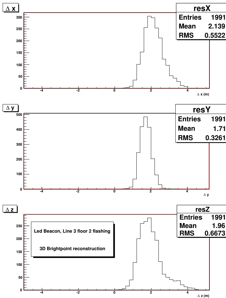
FIG. 5.3 – Différence entre la position de la balise et celle retrouvée par le système de positionnement. Dans les coordonnées X ( en haut ), Y ( au milieu ) et Z ( en bas ).
