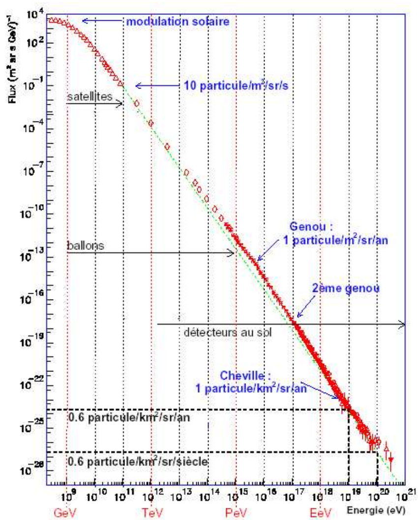
FIG. 1.1 – Spectre de rayons cosmiques
