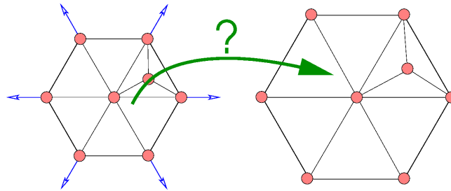
FIG. 3.2.: Expérience d'un hexagone maillé et uniformément gonflé.
