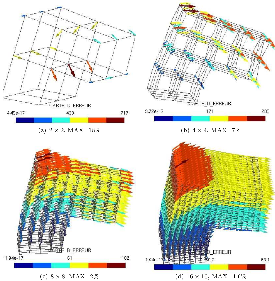
FIG. 3.51.: Cartographie des erreurs sur l'expérience du L pour différentes résolutions : plus la résolution est fine, moins l'erreur est grande.
