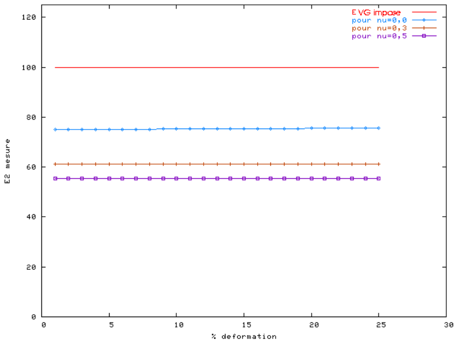
FIG. 3.10: Mesures du module de Young E_2 pour différentes valeurs de \nu_{VG} imposées, et pour E_{VG} = 100MPa.m imposé. On observe une erreur du module de Young effectif par rapport à celui imposé ainsi qu'une dépendance à \nu_{VG} .
