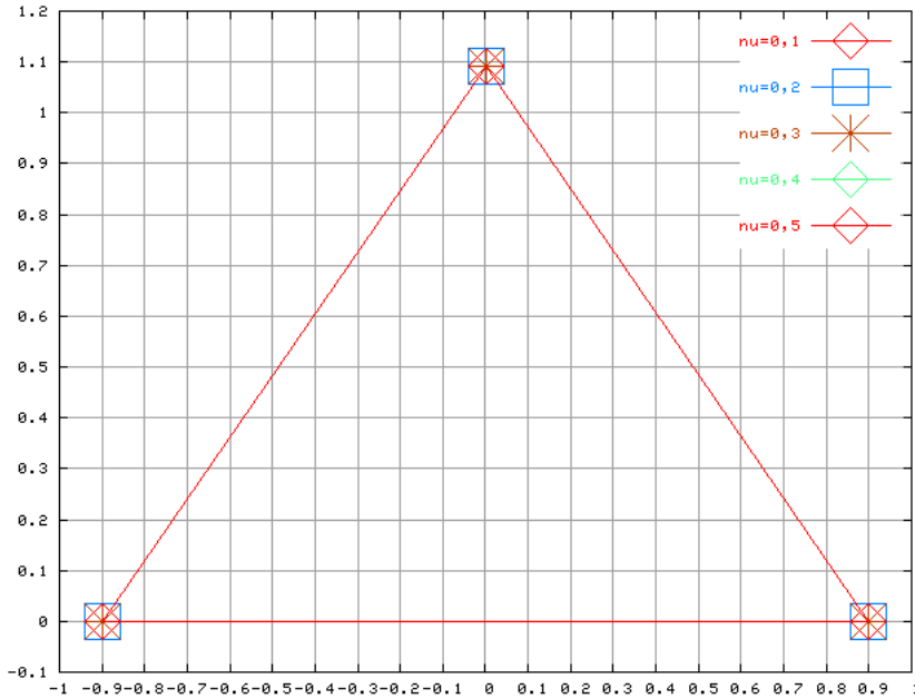
FIG. 3.8.: Résultats superposés des expériences de compression des triangles de Van Gelder paramétrés avec différentes valeurs de \nu : quelque soit la valeur de \nu les triangles réagissent de la même façon à la compression imposée.
