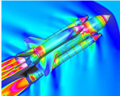
(a) Modèle de contraintes survenant au décollage de la navette spatiale (d'après NASA)
