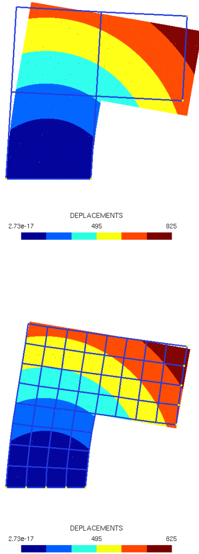
FIG. 3.32.: Superposition du résultat obtenu avec Code Aster pour un maillage fin (en couleur) sur les résultats obtenus avec notre modèle (arêtes) pour les résolutions 1 \times 1 et 4 \times 4
