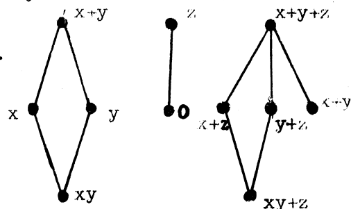
Treillis des \sum Y_1 Treillis Sup demi-des \sum Z_1 treillis des \sum Y_1 + \sum Z_1
