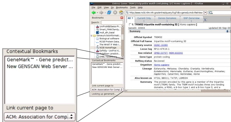
FIG. 3.15: PageLinker
