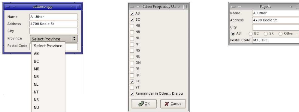
FIG. 3.10: Exemple de substitution d'interface : application originale, dialogue permettant le choix des éléments de la liste à conserver et application personnalisée
