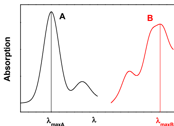
Fig. 1.1 : Équilibre photochromique entre deux espèces A et B ; spectre d'absorption de A (noir) et B (rouge).
