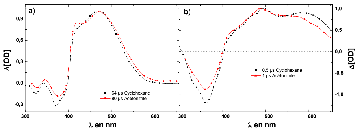
Fig. 4.20 : Spectres d'absorption transitoire obtenus dans le cyclohexane (noir) et dans l'acétonitrile (rouge), pour des retards de a) 64 et 80 μs et b) 0,5 et 1 μs.
