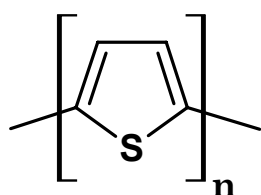
Fig. 2.1 : Structure des \alpha -oligothiophène ( nT ).
