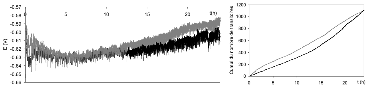
Figure IV.17: Exemple d'essais de reproductibilité en galvanostatique sur le 7449 T651 TR ; à gauche les évolutions du potentiel au cours de l'essai ; à droite les cumuls de transitoires supérieures à 2mV
