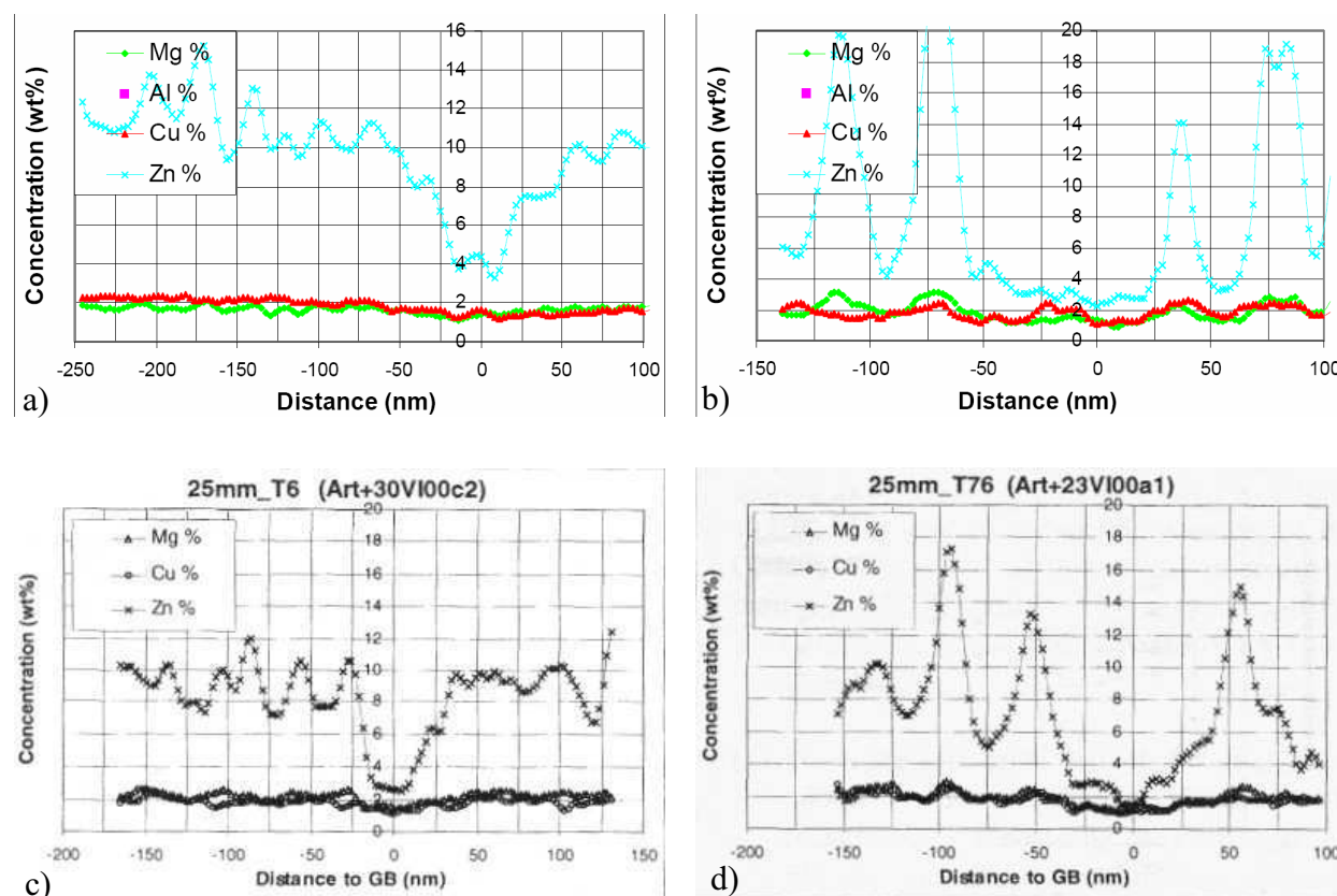
Figure 1.25 : Profils de concentration en soluté, traversant un joint de grain du 7449 des états T6 et T7 : a) et b) [Tanaka, 2002] ; c) et d) [Bellenger, 2002]
