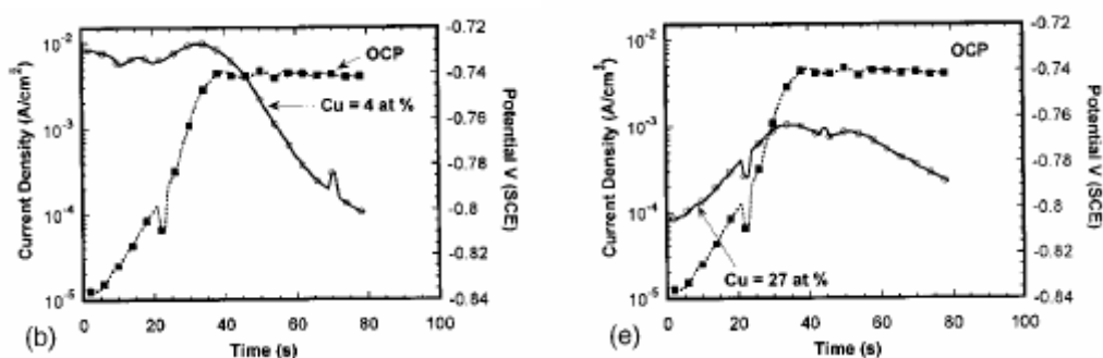
Figure I.26 : Evolution de la densité de courant de dissolution en fonction du temps des phases Mg(Zn,Cu,Al)_2 , représentatives des précipités intergranulaires, dans un milieu aéré 0.5MNaCl, lorsqu'on leur impose le potentiel, correspondant au potentiel d'abandon mesuré sur le 7150 T6 dans cette même solution.
