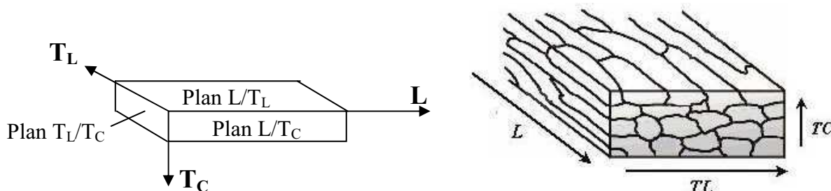
Figure II.1 : Définition des directions principales de la tôle
