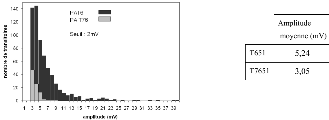
Figure IV.16: Distributions en amplitude des transitoires pour le PA T651 et T7651 pour un seuil de détection de 2 mV
