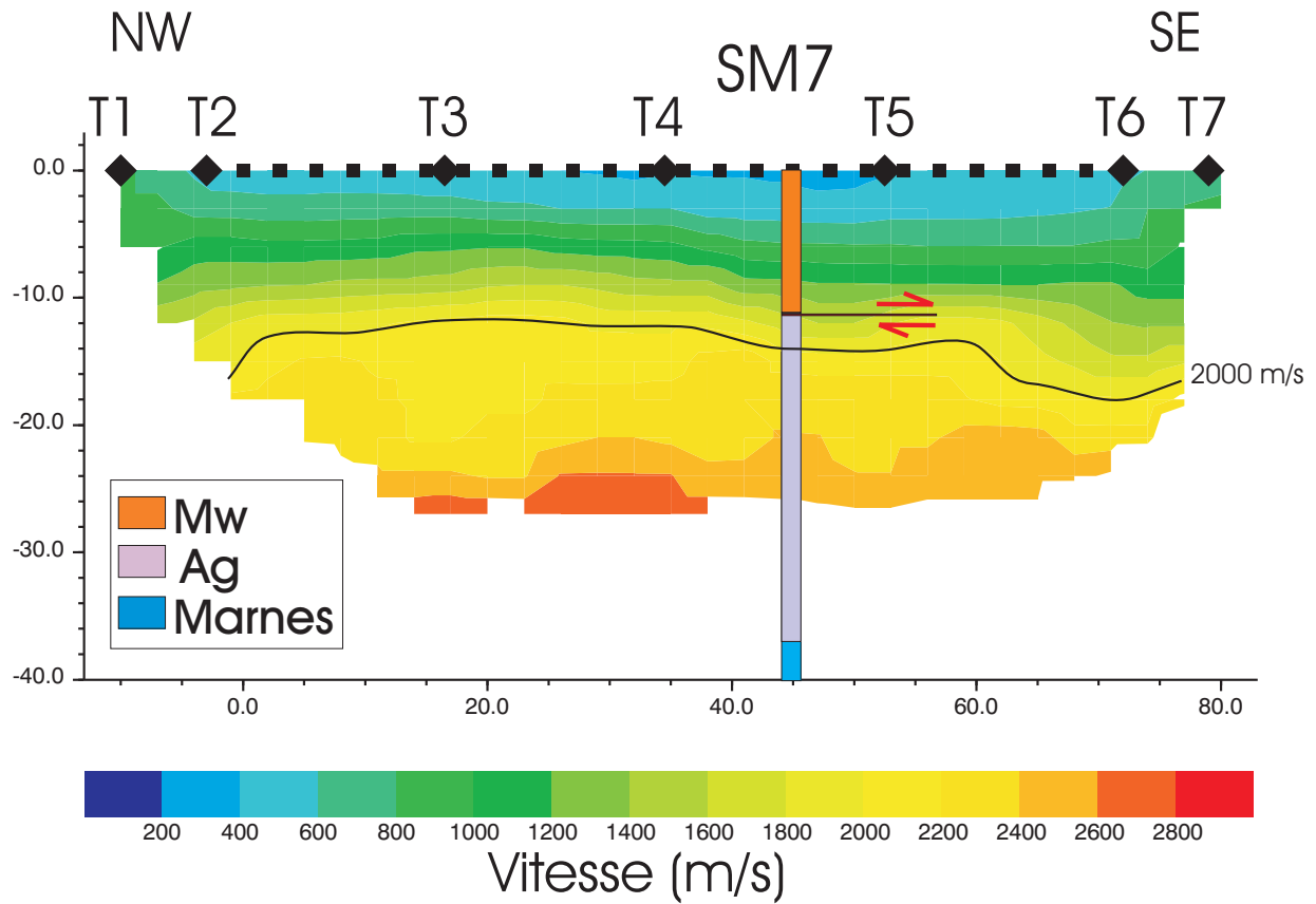
FIG. 8.11 – Tomographie sismique du glissement de Léaz le long d'un profil longitudinal au mouvement (PS2)
