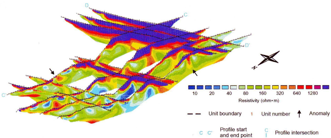
FIG. 1.3 – Représentation 3D de tomographies électriques 2D mesurées sur un glissement dans les argiles et sables (British Columbia, Canada), d'après Bichler et al. (2004)
