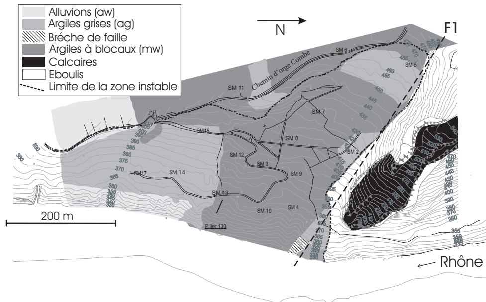
FIG. 8.3 – Carte topologique montrant les limites du glissement de Léaz ainsi que les formations géologiques, la localisation des sondages mécaniques et de la coupe géologique (a-a') présentée à la figure 8.4
