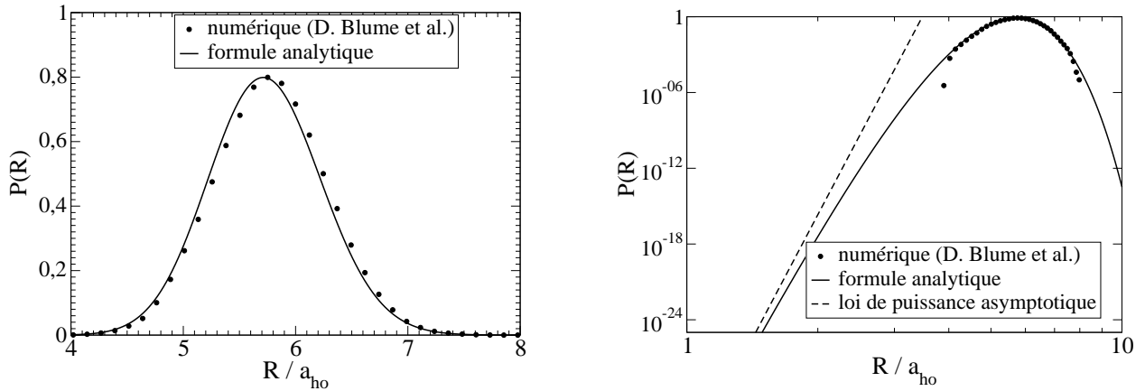
FIG. 8 – Mêmes quantités que la Figure 6, pour l'état fondamental à N = 17 particules. Les valeurs numériques sont obtenues par une méthode Monte-Carlo à nœuds fixés, l'énergie obtenue étant E = 34.64(12)\hbar\omega [28].
