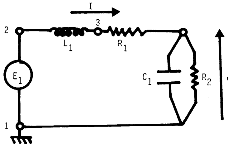
FIG. II-7 Exemple de circuit électrique
