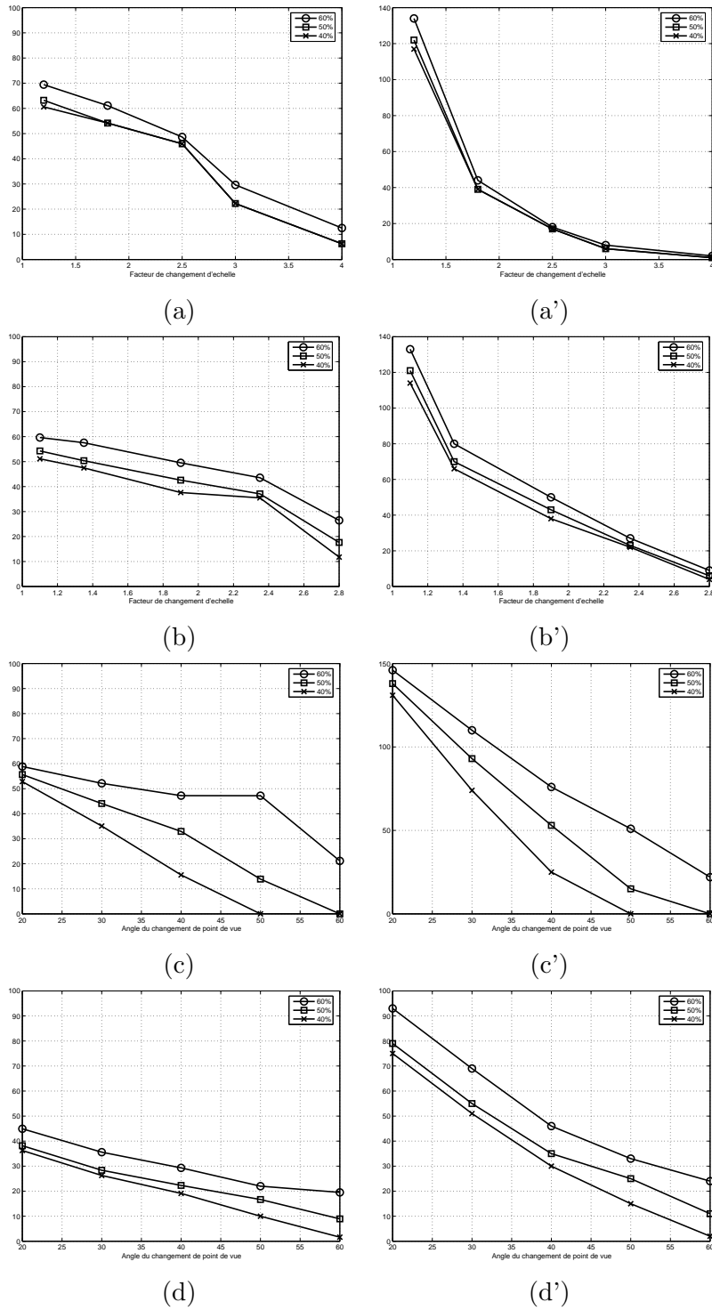
FIG. A.8 – Performance du détecteur ML (points d'intérêt : cercles ( x^*, y^*, S^* )). Score de répétabilité et nombre de correspondances pour les séquences : (a) ZoomRotation1, (b) ZoomRotation2, (c) Viewpoint1, (d) Viewpoint2.
