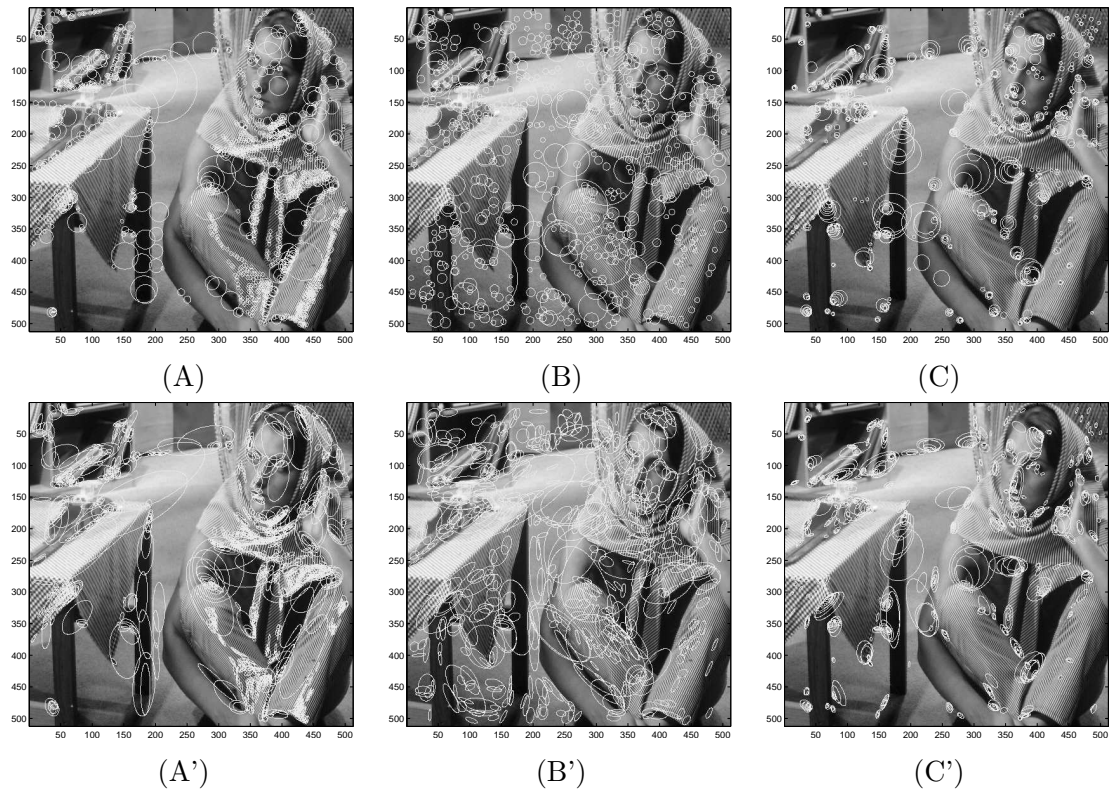
FIG. 7.5 – Application de détecteurs classiques en vision par ordinateur (A, A') Laplacien de Gaussienne (LoG); (B, B') Différence de Gaussienne (DoG); (C, C') Harris-Laplace (HL); (A, B, C) Points d'intérêts (x^*, y^*, s^*) ; (A', B', C') Régions affines (x^*, y^*, s^*, \Sigma^*) .
