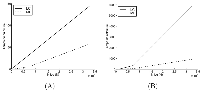
FIG. 5.6 – Temps de calcul effectif en fonction de N \log N , pour un carré en (A), et pour un carré bruité en (B) (les images étant de taille n \times n , la taille des données vaut N = n^2 ).
