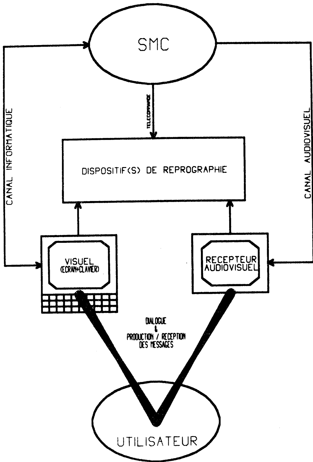
Figure 15: LE POSTE D'ACCES STANDARD (dit aussi "POSTE DE TRAVAIL")
