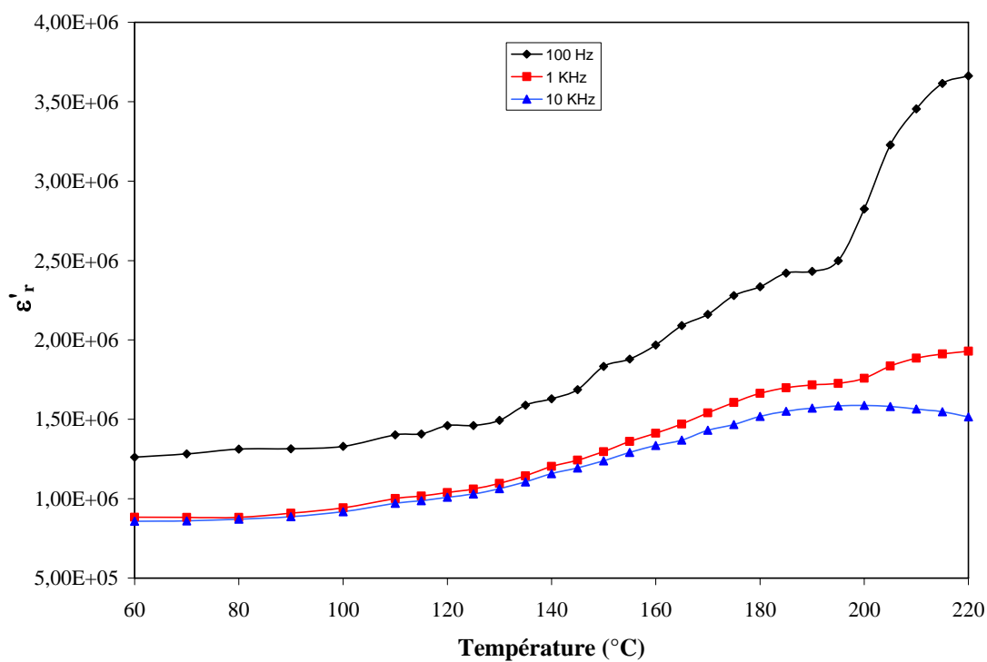
Annexe III-6 : Variation thermique de \epsilon'_t d'une céramique de \text{Sr}_{1,6}\text{Ca}_{0,4}\text{KNb}_5\text{O}_{15} obtenue par voie solide classique.
