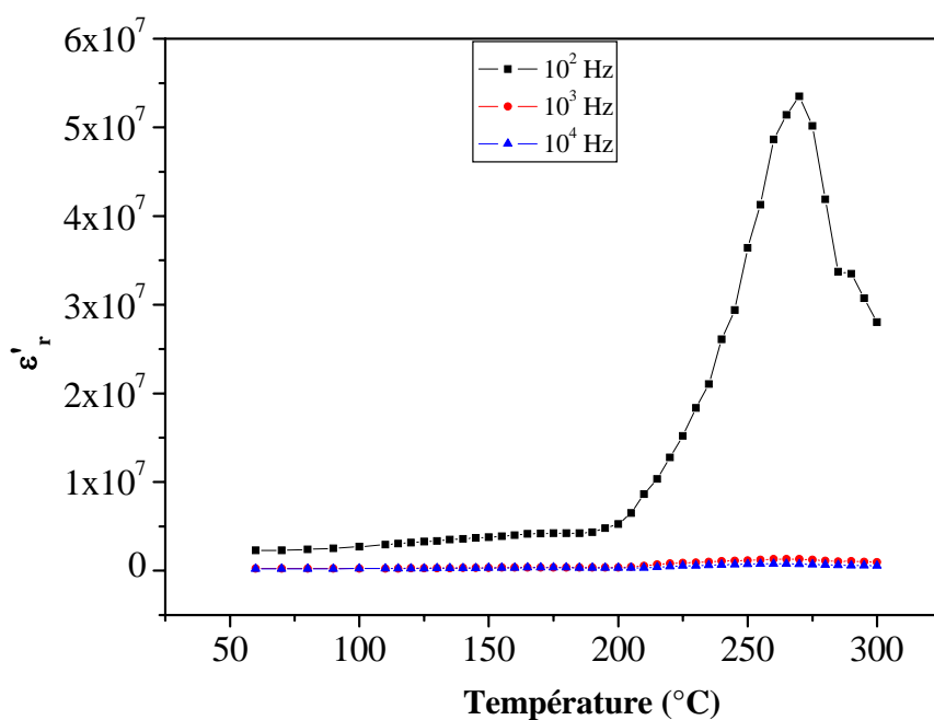
Annexe III-5 : Variation thermique de \epsilon'_t du SKN obtenu par voie solide classique \text{Sr}_{1,8}\text{Ca}_{0,2}\text{KNb}_5\text{O}_{15} .
