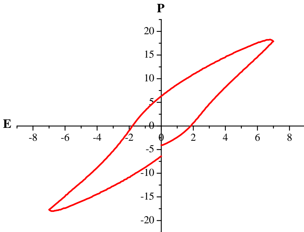
Figure 10 : Cycle d'hystérésis P(V) mesuré sur un condensateur RuO 2 /SBT/Pt.
