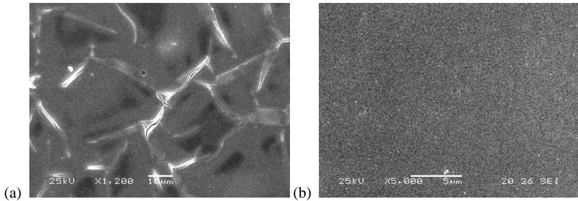
Figure 9 : Micrographies MEB des dépôts de RuO 2 sur BNN (a) et SBT (b).
