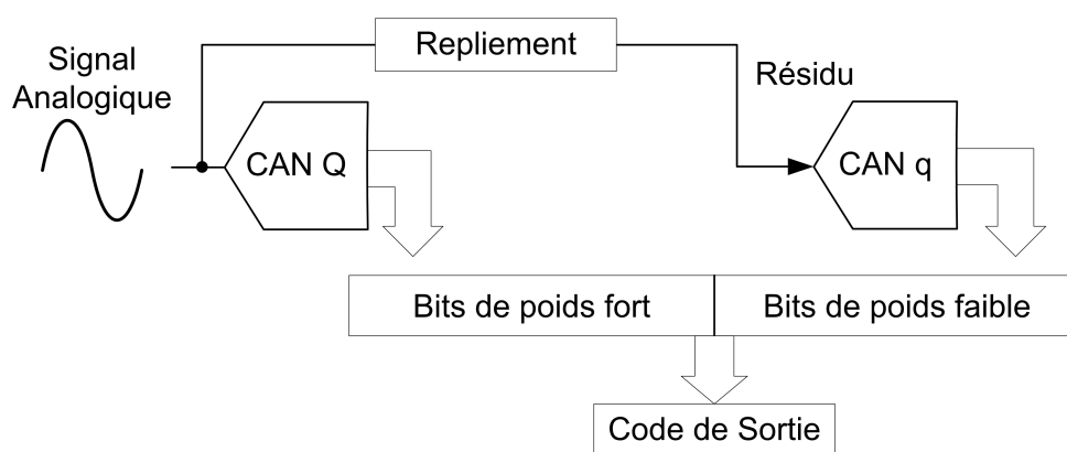
FIG. 1.15 – Principe du Convertisseur à Repliement
