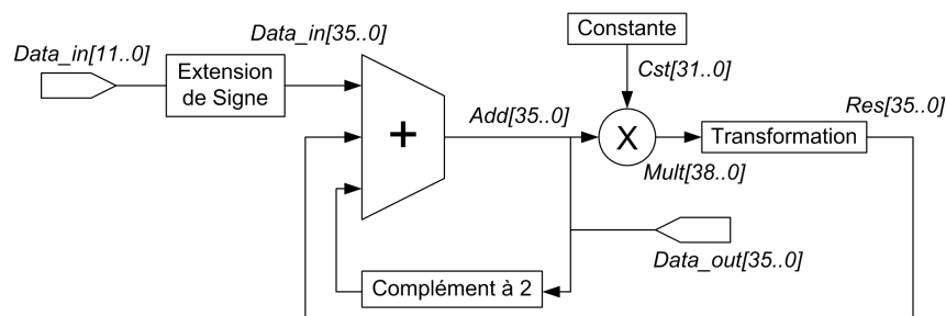
FIG. 5.20 – Architecture de l'implantation de l'algorithme de Goertzel
