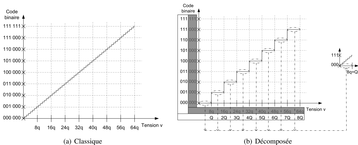
FIG. 1.14 – Fonction de transfert d'un pipeline par troncature
