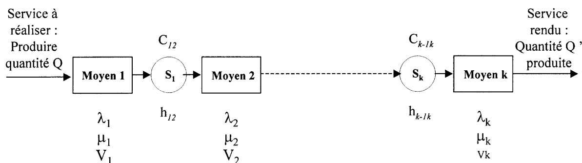
Figure 2.1 : Ligne composée de « n » moyens séparés par un stock intermédiaire
