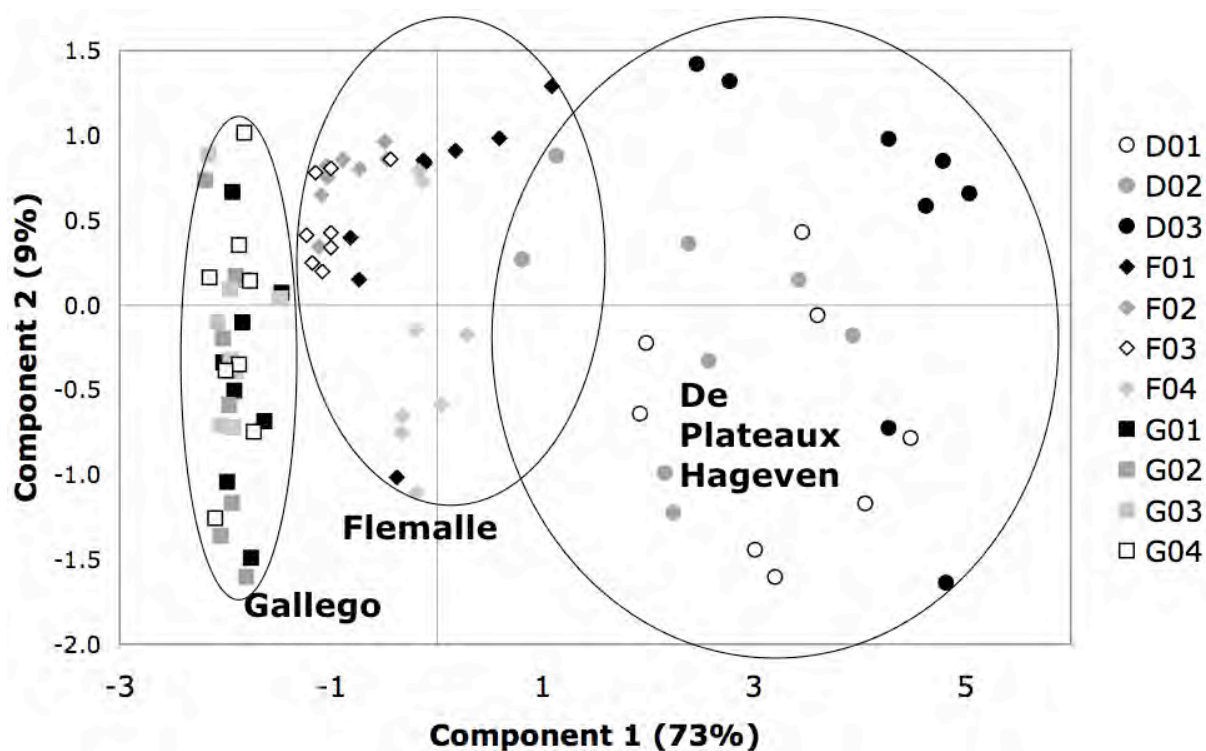
Figure 77 : Représentation des observations de l'ACP effectuée sur les concentrations dissoutes en ETM après 0, 14, 28 et 63 jours d'incubation pour les 11 sols étudiés soumis aux 8 expériences non centrales.
