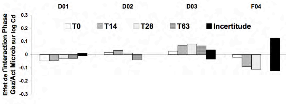
Figure 61 : Effets de l'interaction « Composition de la phase gazeuse/Activité microbienne » sur la solubilisation de Cd des échantillons de sol.
