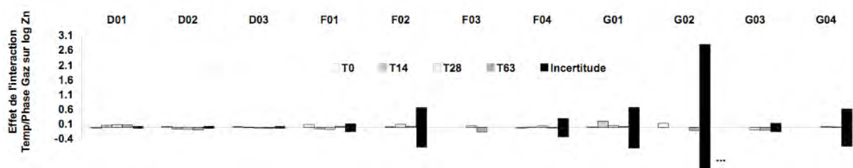
Figure 53 : Effets de l'interaction « Température/Composition de la phase gazeuse » sur la solubilisation de Zn des échantillons de sol. L'incertitude dans le domaine négatif de l'axe est tronqué pour G02.
