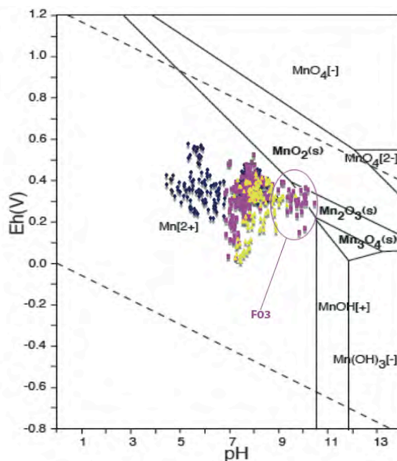
Figure 90 : Estimation de la spéciation de Mn dans le système Mn-O-H ( 10^{-10} mol.kg -1 et conditions standards de température et pression, Takeno, 2005) d'après le pH et Eh mesurés pour les échantillons De Plateaux-Hageven (bleu), Flémalle (rose) et Gallego (jaune).
