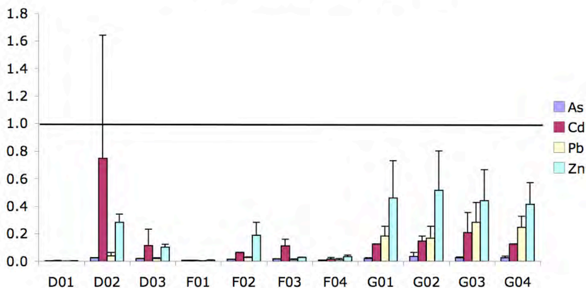
Figure 133 : Facteurs de bioaccumulation de As, Cd, Pb et Zn par le ray grass au niveau des feuilles pour les 11 sols étudiés. La barre d'erreur correspond à l'écart-type obtenu à partir des expériences en triplicat.
