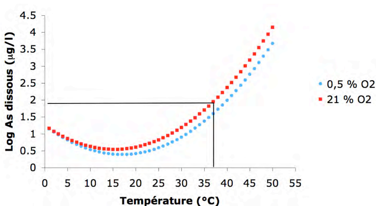
Figure 106 : Log As dissous en fonction de la température selon le modèle du Tableau 44 pour une faible et une forte concentration en oxygène
