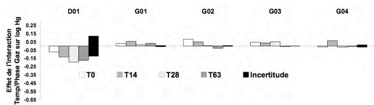
Figure 74 : Effets de l'interaction « Température/Composition de la phase gazeuse » sur la solubilisation de Hg des échantillons de sol.
