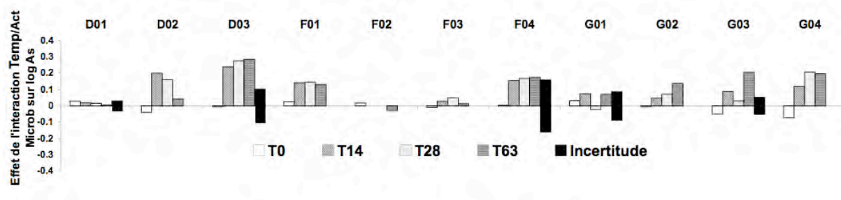
Figure 49 : Effets de l'interaction « Température/Activité microbienne » sur la solubilisation de As des échantillons de sol.
