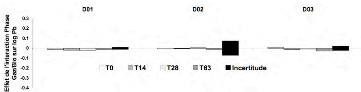
Figure 68 : Effets de l'interaction « Composition de la phase gazeuse/Activité microbienne » sur la solubilisation de Pb des échantillons de sol.
