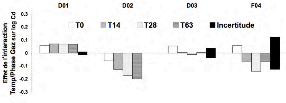
Figure 60 : Effets de l'interaction « Température/Composition de la phase gazeuse » sur la solubilisation de Cd des échantillons de sol.
