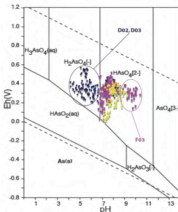
Figure 100 : Estimation de la spéciation de As dans le système As-O-H ( 10^{-10} mol.kg -1 et conditions standards de température et pression, Takeno, 2005) d'après le pH et Eh mesurés pour les échantillons De Plateaux-Hageven (bleu), Flémalle (rose) et Gallego (jaune).
