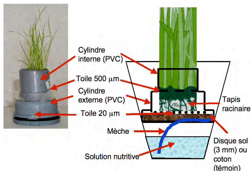
Figure 129 : Schématisation de l'étape finale de culture sur sol (adapté de El-azab, 2005).
