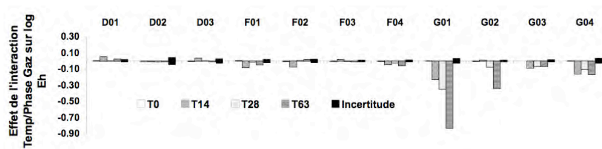
Figure 98 : Effet de l'interaction entre « Température » et « Composition de la phase gazeuse » sur Eh.
