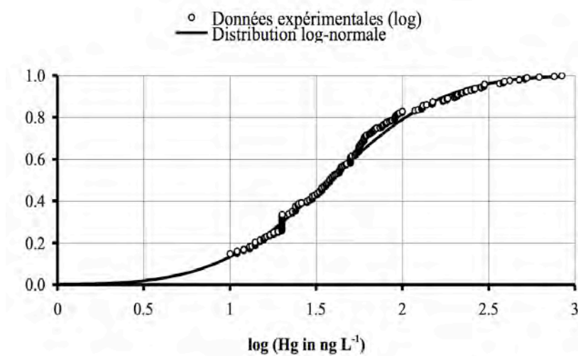
Figure 205 : Distribution (entre 0 et 1) du logarithme des concentrations aqueuses en Hg pour D01, G01, G02, G03, G04 et SG1 (286 observations) en comparaison à une distribution log-normale.
