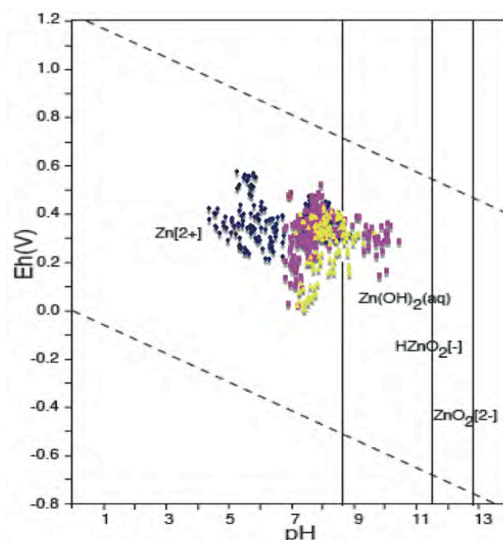
Figure 99 : Estimation de la spéciation de Zn dans le système Zn-O-H ( 10^{-10} mol.kg -1 et conditions standards de température et pression, Takeno, 2005) d'après le pH et Eh mesurés pour les échantillons De Plateaux-Hageven (bleu), Flémalle (rose) et Gallego (jaune).
