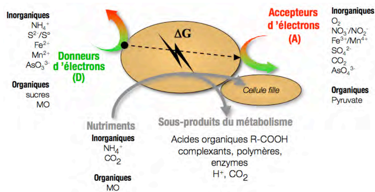
Figure 6 : Métabolisme d'une bactérie (modifié d'après Deneux-Mustin et al., 2003).
