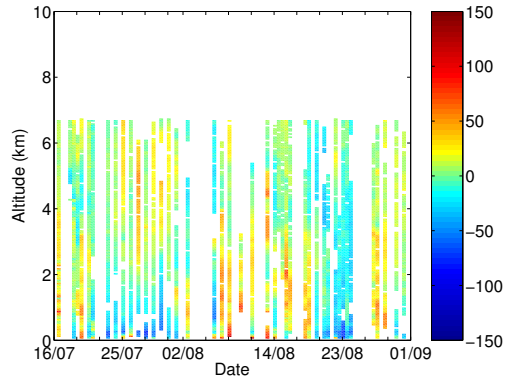
(b) Anomalie de CO à Paris
