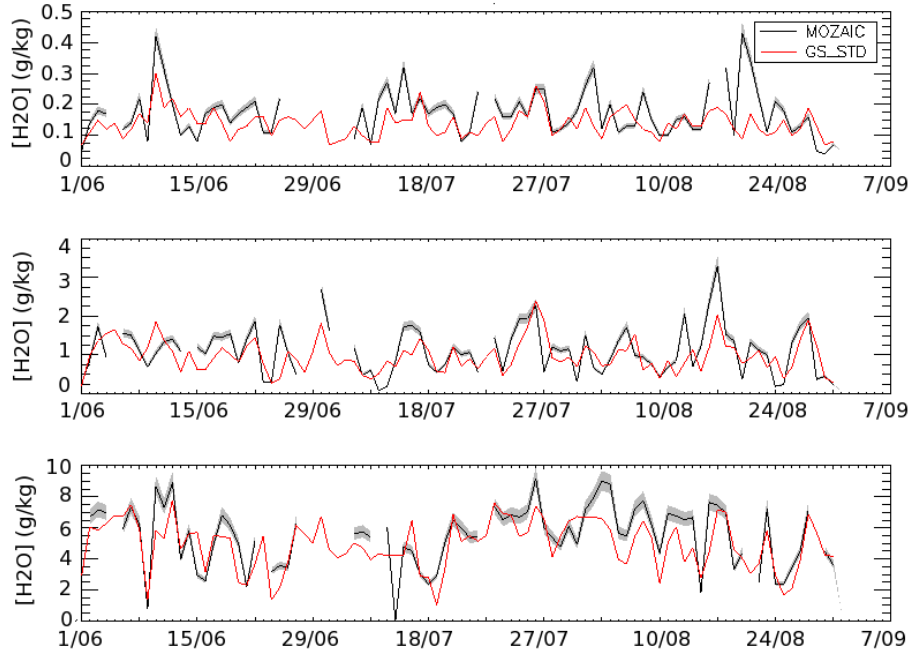
FIG. 3.2 – Evolution de la vapeur d’eau (en g/kg) à Francfort du 1 er Juin au 31 Août pour les niveaux de pression (de bas en haut : 800 hPa, 500 hPa et 300 hPa). Les valeurs pour MOZAIC sont représentées en noir et en rouge pour GEOS-Chem. La zone grisée présente l’erreur de mesure.
