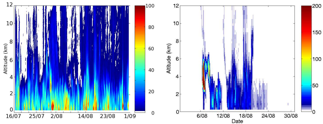
(c) CO européen à Vienne
