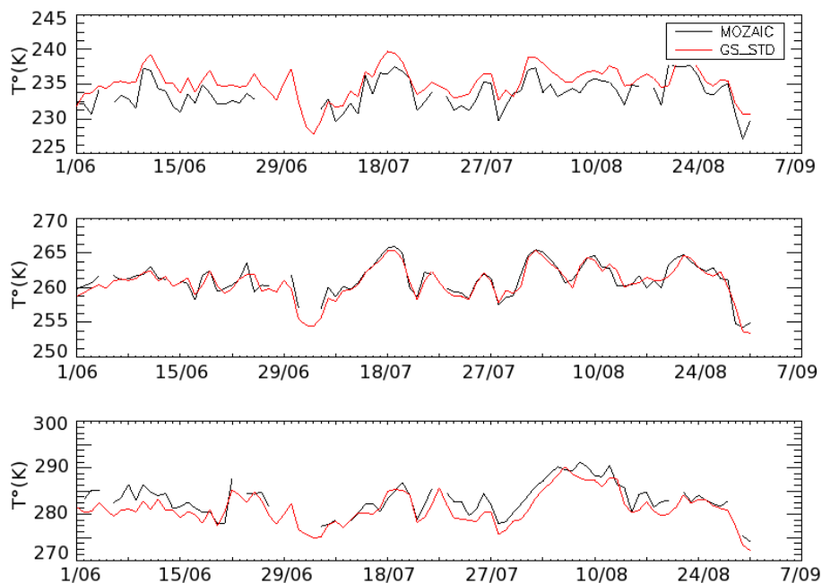
FIG. 3.1 – Evolution de la température (en K) à Francfort du 1 er Juin au 31 Août pour les niveaux de pression (de bas en haut : 800 hPa, 500 hPa et 300 hPa). La température MOZAIIC est représentée en noir et la température GEOS-Chem en rouge.
