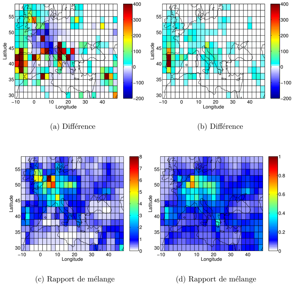
FIG. 3.15 – En haut : Différence des rapports de mélange des \text{NO}_x (en pptv) moyennée sur la période caniculaire (2-14 Août) entre la simulation EMX3 et la simulation STD pour les niveaux 1 (sol) et 5 (2000 m) du modèle (de gauche à droite).
