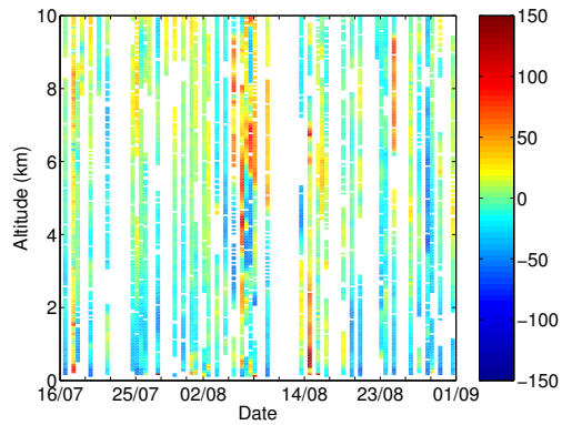
(d) Anomalie de CO à Vienne
