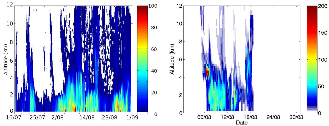
(a) CO européen à Paris
