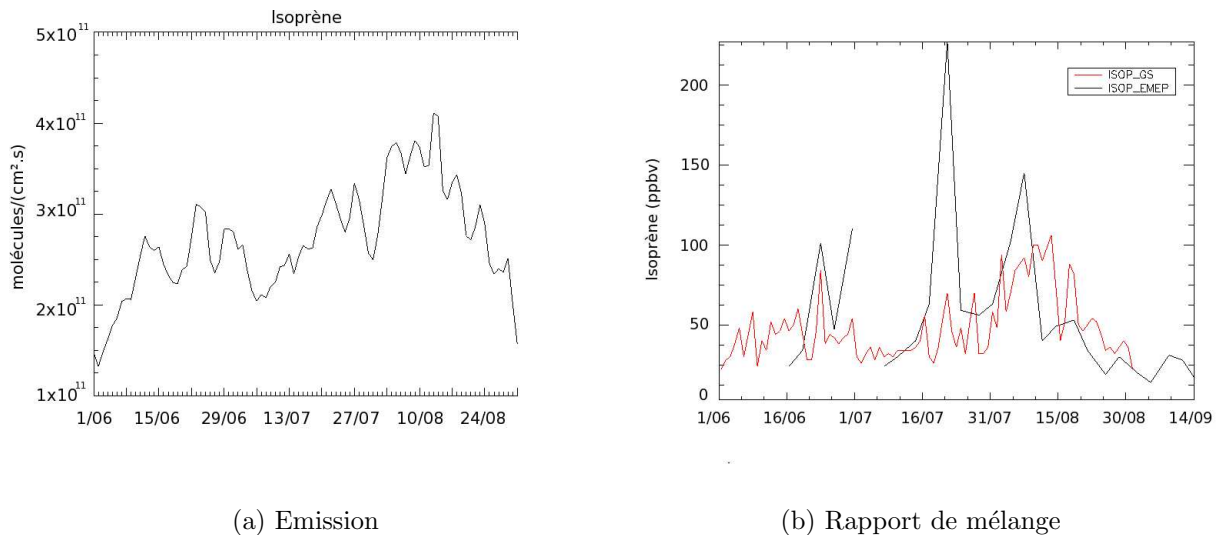
FIG. 3.9 – (a) Evolution temporelle des émissions d’isoprène moyennées sur l’Europe du 1 er Juin au 31 Août ( \text{molécules} \cdot \text{cm}^{-2} \cdot \text{s}^{-1} ). (b) Evolution temporelle du rapport de mélange de l’isoprène modélisé (rouge) et mesuré (noir) en pptv à Schmüke.
