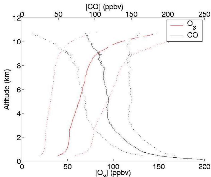
FIG. 1.3 – Profil vertical climatologique (ligne continue) du rapport de mélange (en ppbv) de l’ozone (en rouge) et du CO (en noir) à Francfort selon MOZAIC. La déviation standard est représentée en pointillée.
