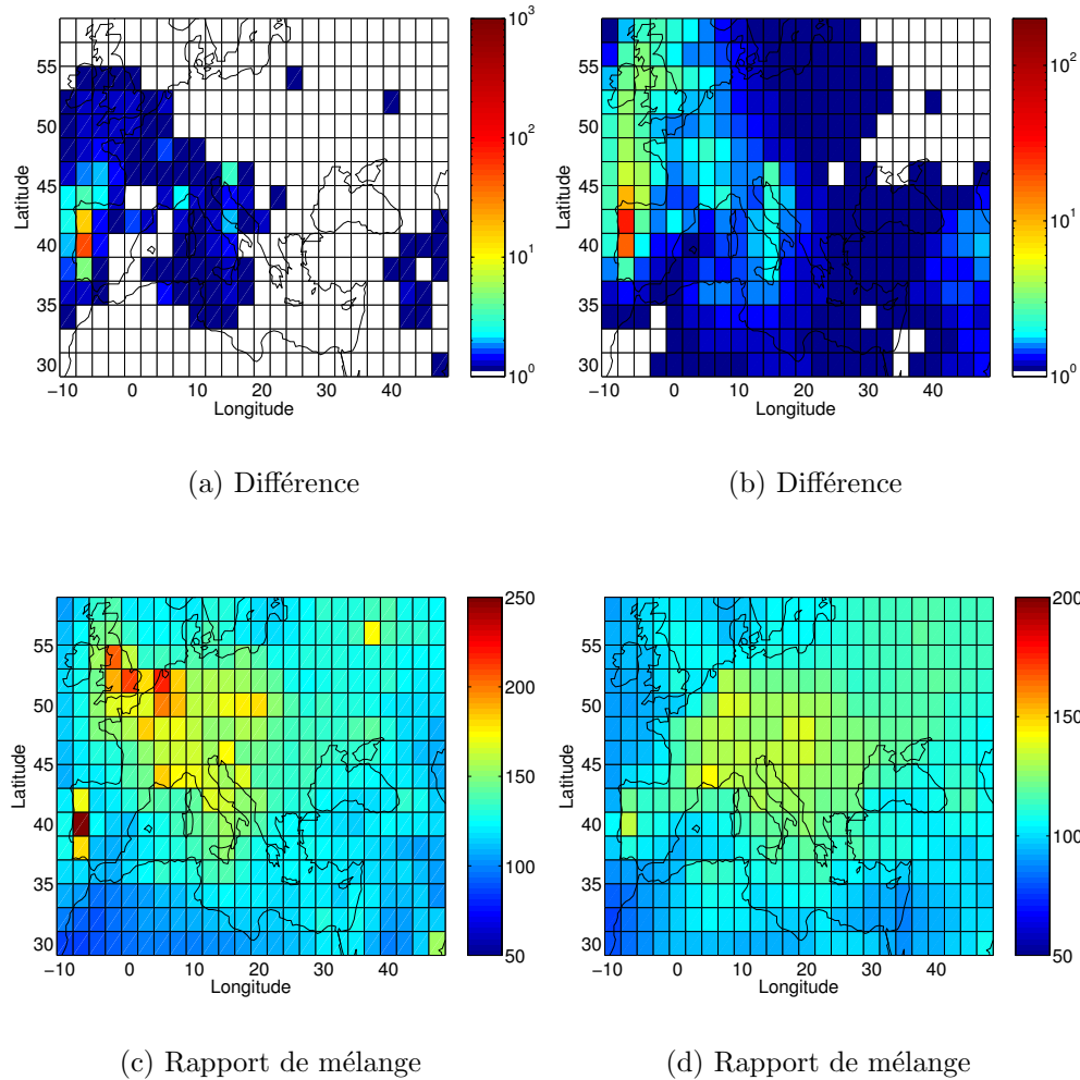
FIG. 3.16 – En haut : Différence des rapports de mélange de CO (en ppbv) moyennée sur la période caniculaire (2-14 Août) entre la simulation EMX3 et la simulation STD pour les niveaux 1 (sol) et 5 (2000 m) du modèle (de gauche à droite).
