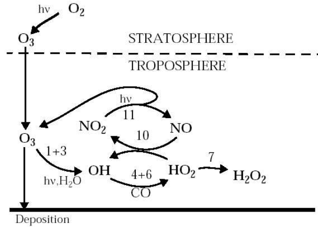
FIG. 1.2 – Principaux puits et sources de l’ozone troposphérique (d’après Jacob, 1999 [38]).
