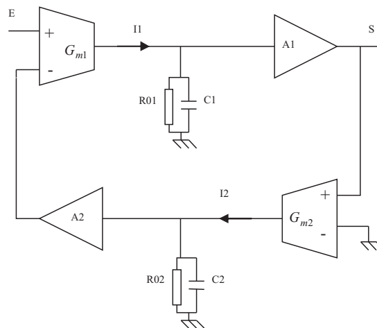
FIG. C.2 Modèle du résonateur Gm-C
