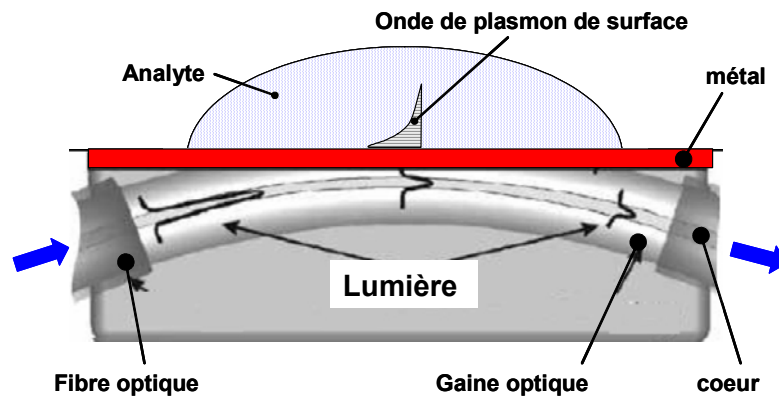
Figure II.5 : Illustration d'un CFO ayant sa zone sensible polie sur un seul côté de la fibre optique qui est fixée dans un bloc de silice [15].
