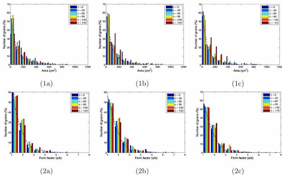
Figure 45B : Distribution de la taille de grains (1) et du facteur de forme (2) pour différentes sections prélevées suivant les trois directions a) x, b) y, c) z. [St Pierre, 07]
