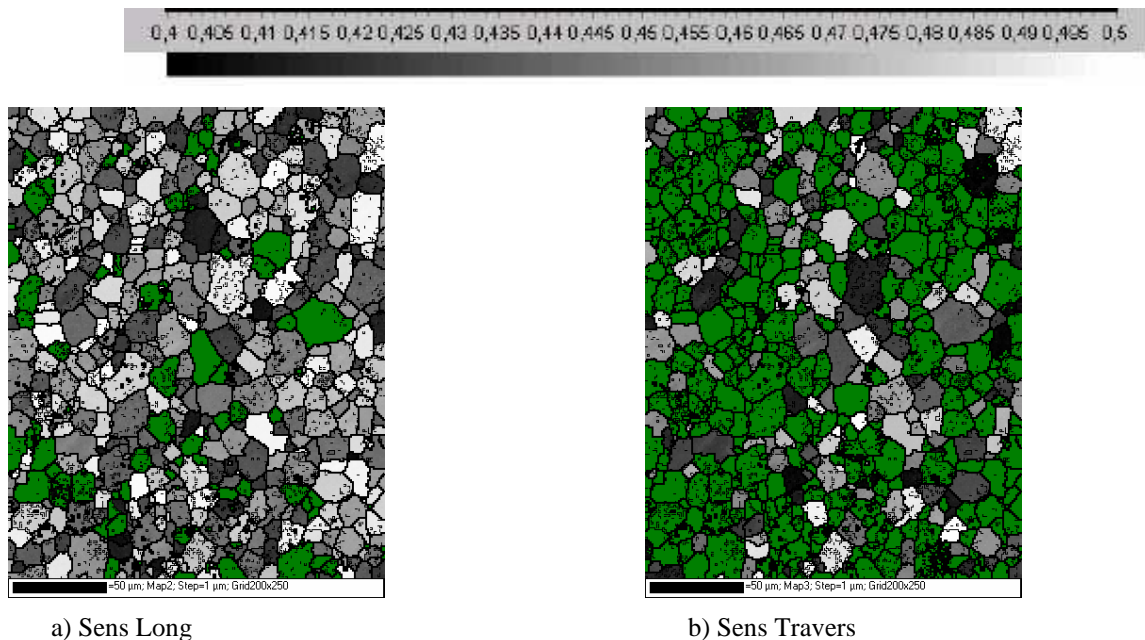
Figure 24 : Visualisation de la répartition des grains « durs » en vert au sein de la microstructure d'un alliage de zirconium grade 702 recrystallisé. Le critère d'écoulement local retenu correspond à 0,4.
