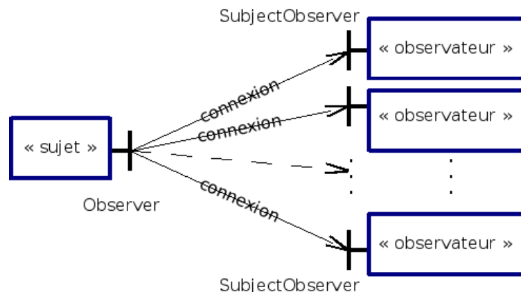
FIGURE 3.14 – illustration du motif d’architecture sujet observateur
