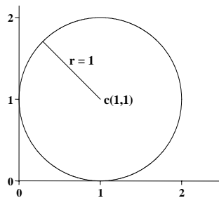
Figure 2 : Représentation du disque \{1+i; 1\}
