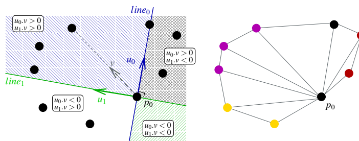
FIG. C.2 – Triangulation d'un contour dans le plan
