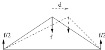
FIG. 2.25 – Couple fantôme.
