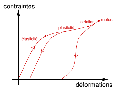
FIG. 2.14 – Matériau plastique
