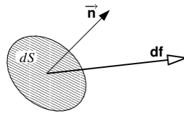
FIG. 2.7 – Force élémentaire
