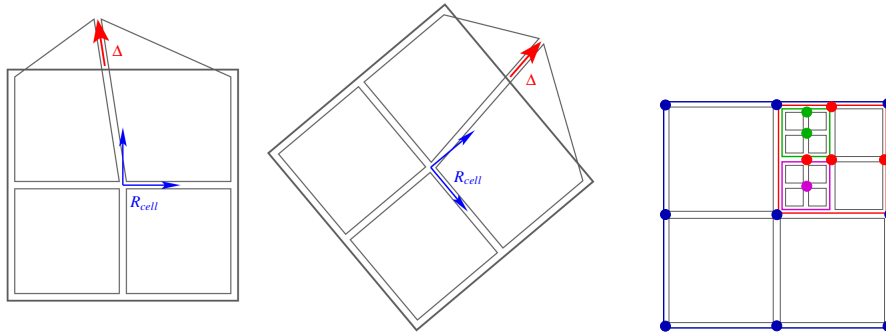
FIG. 5.9 – Prise en compte des grands déplacements hiérarchiques
