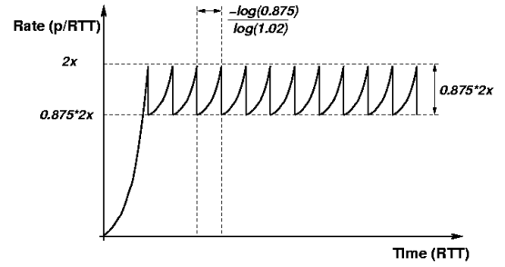
(d) STCP - Large Capacity
