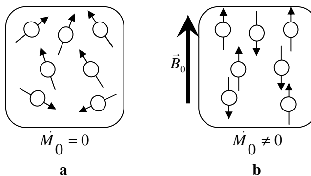
Figure 1-1 : Les spins (ici dans le cas des protons de l'eau où le spin = \frac{1}{2} ) (a) aléatoirement orientés dans l'espace (b) s'alignent en présence d'un champ magnétique B_0 , créant ainsi une aimantation macroscopique M_0 .
