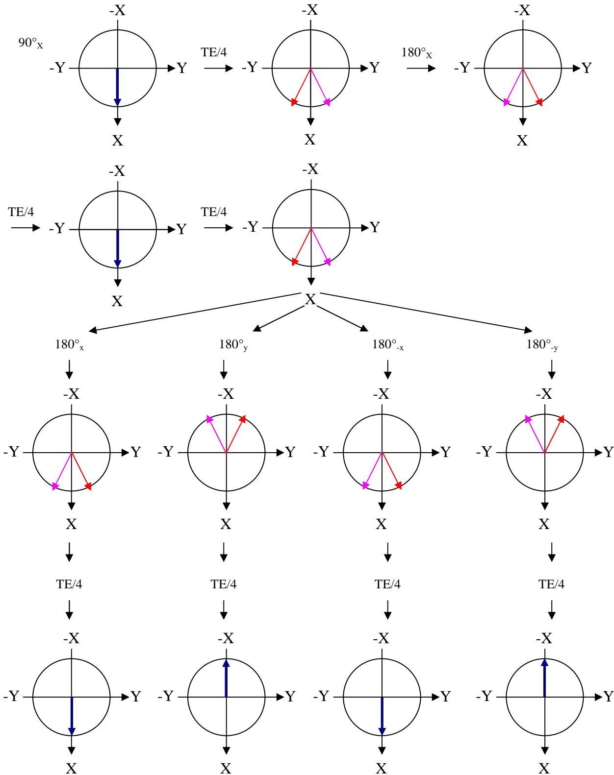
Figure A3-1 : Diagramme vectoriel de l'aimantation du cyclage de phase EXORCYCLE.
