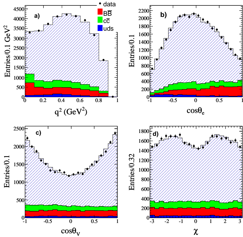
Figure 1: Distributions des valeurs reconstruites des variables cinématiques définissant la désintégration D_s^+ \rightarrow \phi e^+ \nu_e . Les points représentent les données, les histogrammes hachurés correspondent au signal fitting et les histogrammes pleins sont les estimations du bruit de fond obtenues d'après la simulation.
