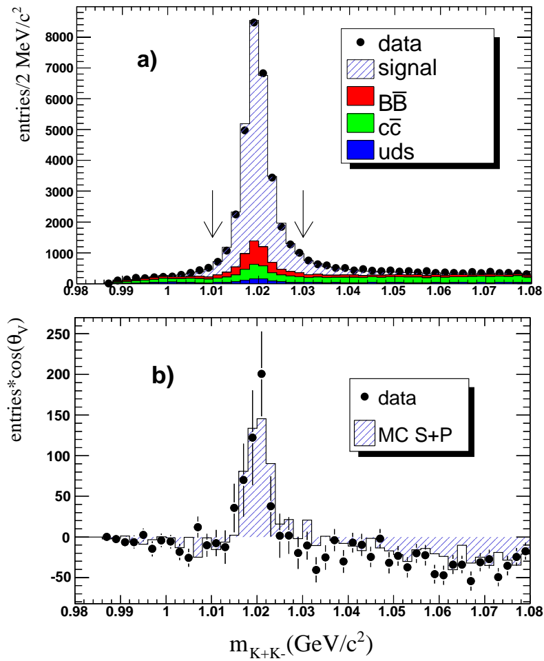
Figure 2: Distributions en masse K^+K^- . a) Comparaison entre les données et la simulation du signal et du bruit de fond. b) Distributions en masse K^+K^- pondérée par \cos\theta_V , les données sont comparées à la simulation dans laquelle une composante d'onde S a été ajoutée.
