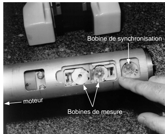
Figure 3.12 - Photographie de la partie de l'équilibre recevant les deux bobines de mesure montées tête-bêche et la bobine de synchronisation.
