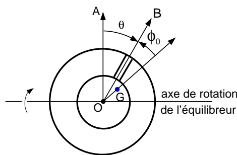
Figure 3.14 - Définitions de \theta et \phi_0 . G représente le centre magnétique de la bobine.
