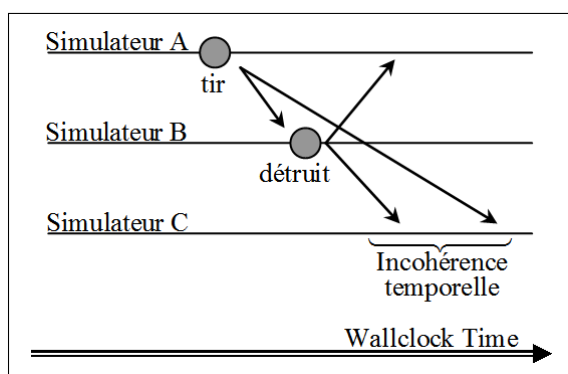
FIGURE 2.3 – Problème d'ordonnancement causal.
