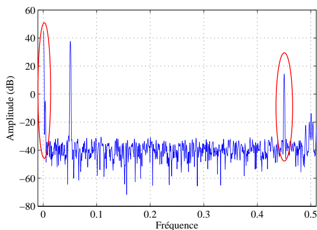
FIG. 6.9 – Spectre de sortie mesuré à la sortie du TIADC avant implémentation de la méthode de correction.
