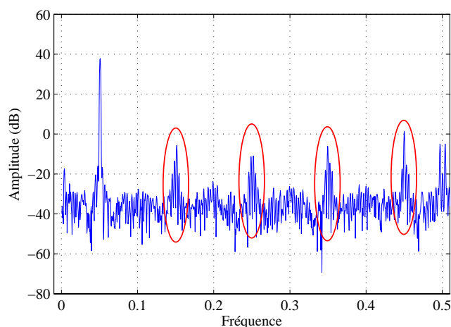
FIG. 6.10 – Spectre de sortie mesuré à la sortie du TIADC après implémentation de la méthode de correction.
