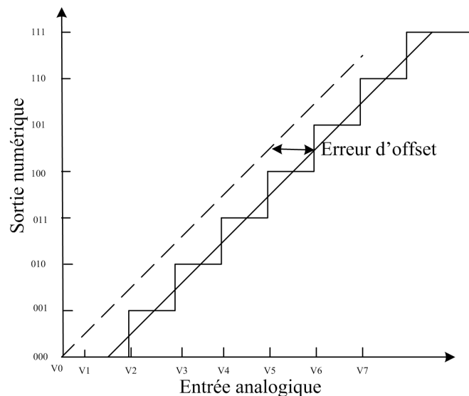
FIG. 2.3 – Erreur d'offset.
