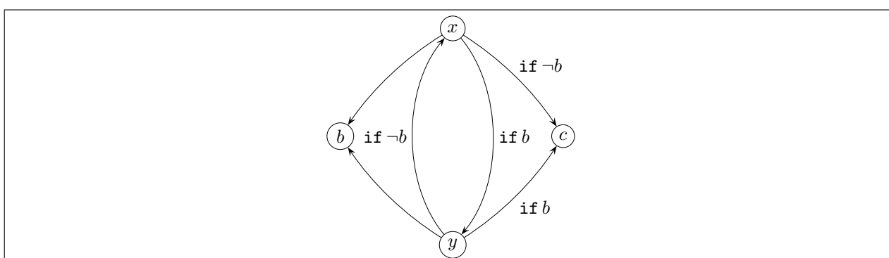
FIG. 1 – Graphe des dépendances des équations (1) à (4).
