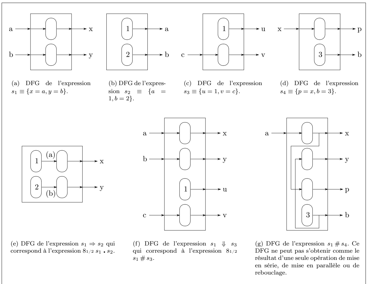
FIG. 7 - Exemple de composition de système dans un style fonctionnel et avec les amalgames.
