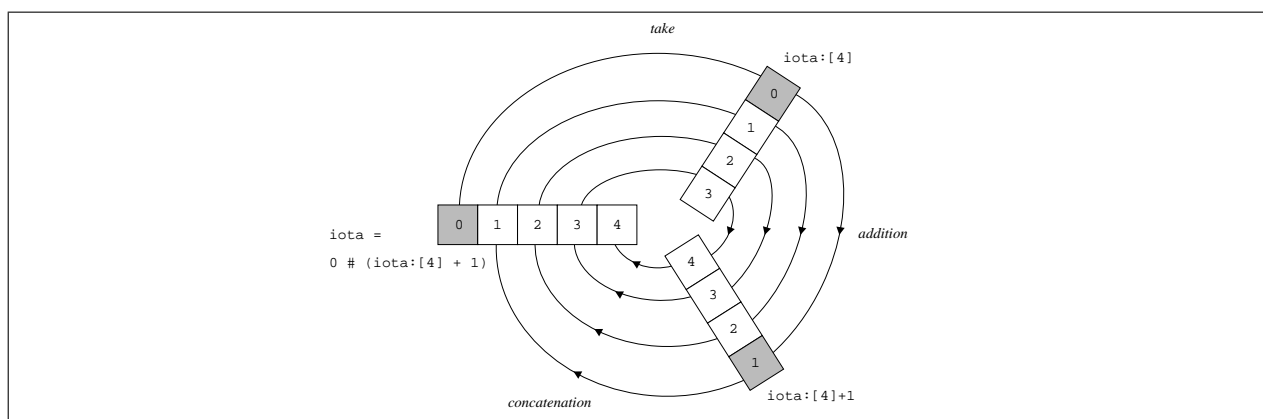
FIG. 5 – Calcul de iota[5] par une méthode de récursion spatiale. L'indice correspond au numéro de génération de la valeur de la collection iota : à l'initialisation, seule la valeur de iota \cdot 0 est connue ; ensuite, par propagation du calcul vers la droite, l'ensemble des valeurs de la collection est calculé.
