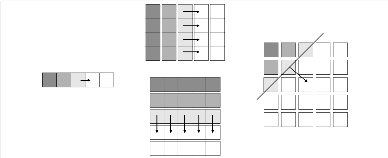
FIG. 5 – Propagation des calculs dans la définition récursive d'un tableau en 8_{1/2} . Le premier schéma illustre la propagation des calculs lors de la résolution d'une définition récursive d'un vecteur, comme par exemple la définition de iota (voir figure 5). Le deuxième schéma illustre une propagation pour un tableau à deux dimensions. Il faut noter que pour chaque axe, la propagation peut se faire de l'index 0 vers les index croissants, ou de la borne supérieure du tableau vers l'index 0. Le troisième schéma montre un processus de calcul qui se propage en diagonale. Il n'est pas possible de définir un tel processus en 8_{1/2} , alors que cela semble être naturel.
