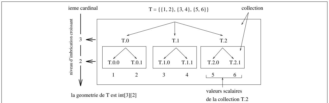
FIG. 1 – La géométrie des collections imbriquées homogènes en 8_{1/2}
