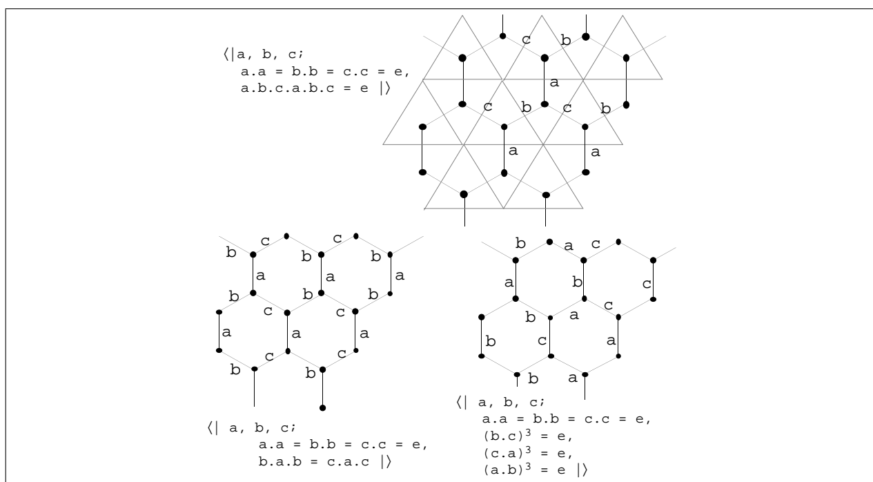
FIG. 6 – Trois exemples de formes à trois voisins. Ces formes ne sont pas abéliennes.
