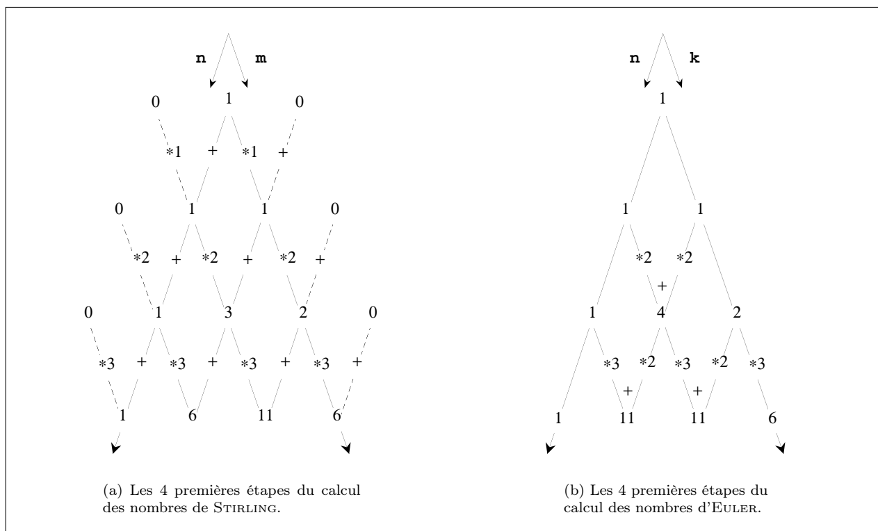
FIG. 1 – Calcul des suites récurrentes par la méthode de Li Shanlan. Exemple du calcul des nombres de Stirling et d'Euler.
