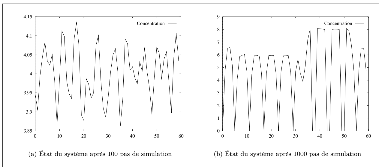
FIG. 2 – Équation de diffusion-réaction dans un tore, d'après A. Turing. Le résultat de la simulation est représenté après 100 pas de temps élémentaires (figure (a)), et après 1000 pas de temps, alors que le phénomène décrit par le système dynamique est stabilisé (figure (b)). La variation constatée peut correspondre à une quantité de colorant et le résultat peut s'interpréter comme des taches périodiquement disposées le long du tore.
