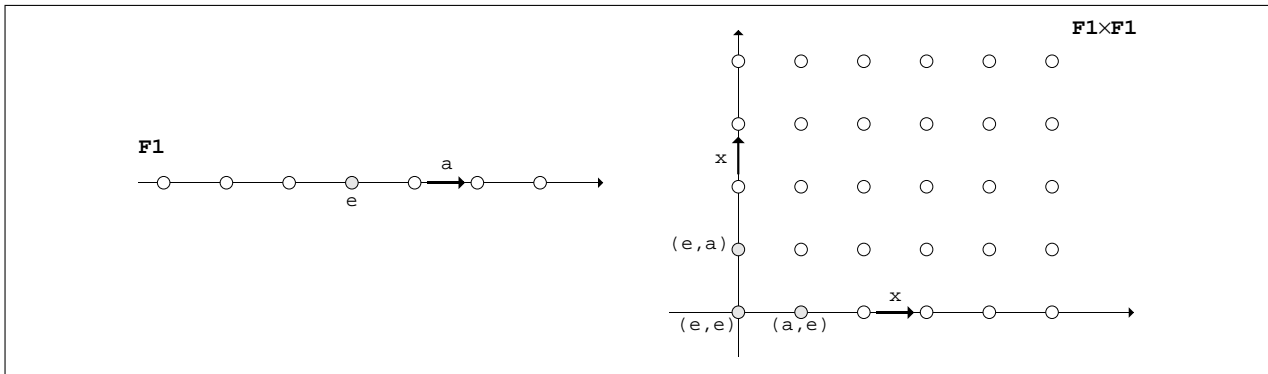
FIG. 9 - Le produit cartésien de deux formes F_1 = \langle a \rangle et F_2 = F_1 \times F_1 .
