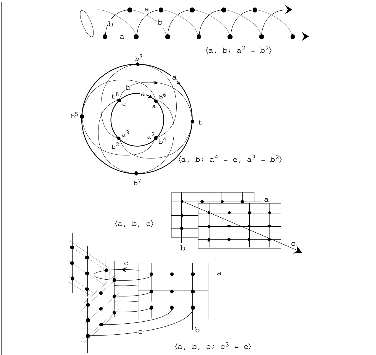
FIG. 5 – Quatre présentations de groupes abéliens et leur graphe Forme(G, S) associé.
