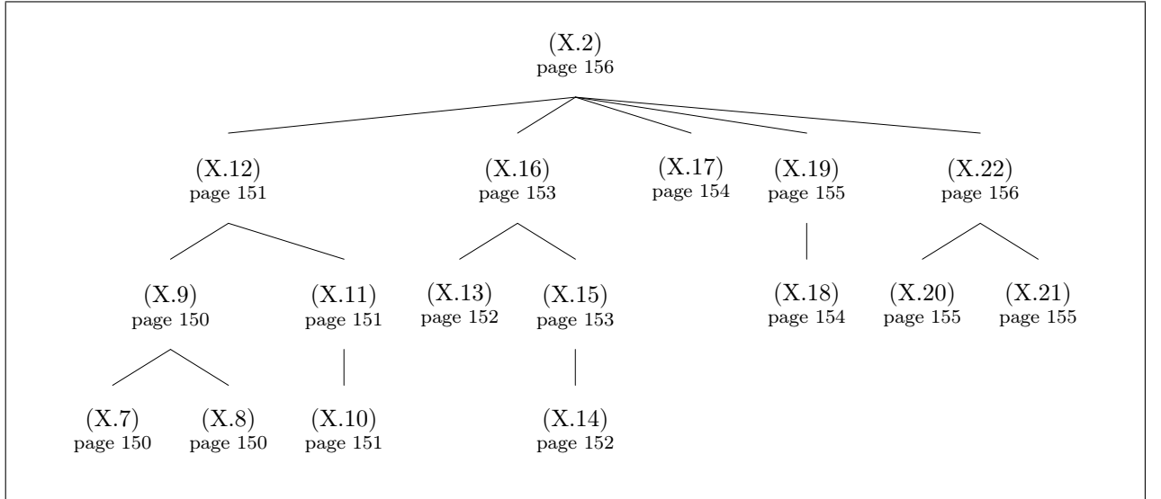
FIG. 3 – Le schéma des dépendances entre les résultats nécessaires à la démonstration du théorème (X.2).
