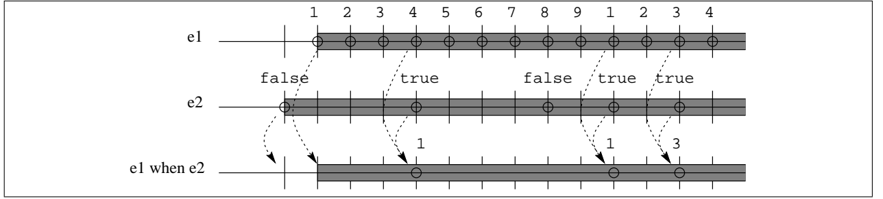
FIG. 3 – Calcul de la valeur de e_1 when e_2 . Le domaine de l'expression est vrai à partir de l'instant où les domaines de e_1 et e_2 sont vrais et où e_2 a une valeur. L'expression possède un top pour chaque top de e_2 où e_2 est vrai, la valeur étant alors celle de e_1 .
