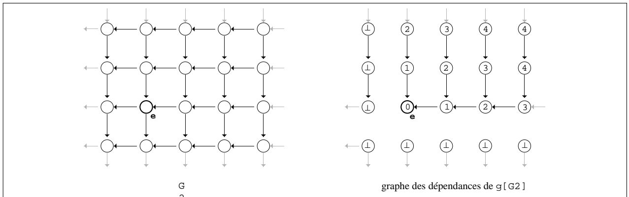
FIG. 2 – Un exemple de forme et de graphe des dépendances associé à un champ g sur cette forme. Le champ g est défini par : g@⟨⟩ = 0 , g@⟨x⟩ = 1 + g.x^{-1} , g = 1 + g.y^{-1} . L'union des graphe des dépendances pour tous les points de la forme ne constitue qu'un sous-graphe de celle-ci.
