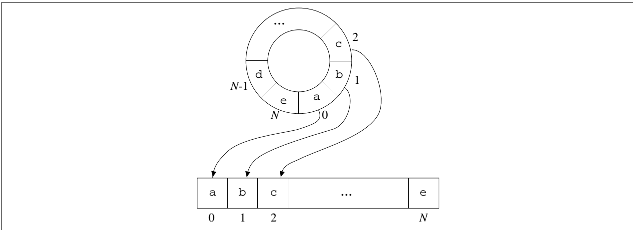
FIG. 1 – Représentation d'une structure torique par un vecteur
