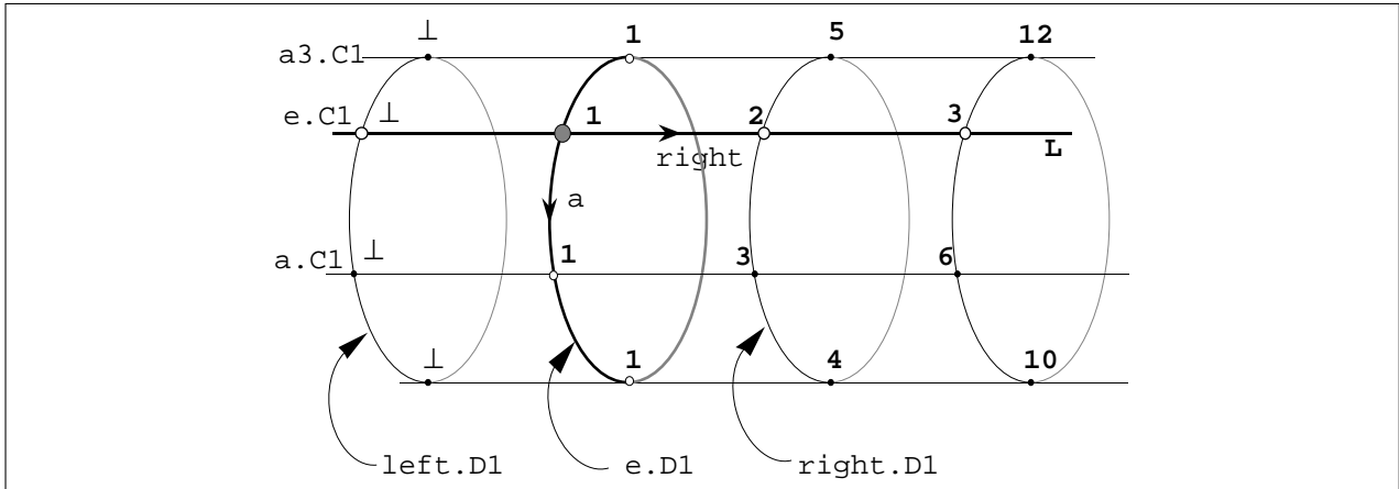
FIG. 1 – Définition d'un champ F sur une partition complexe.
