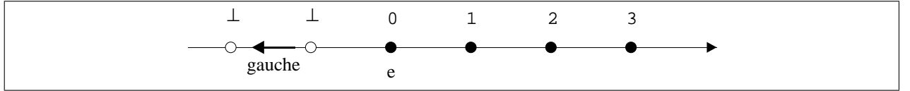
FIG. 15 – Le calcul de iota par un GBF.
