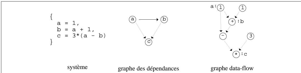
FIG. 3 – Graphe des dépendances et graphe data-flow d'un système.
