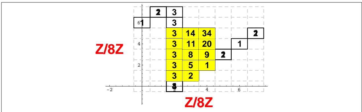
FIG. 2 – Cette figure est un graphique Mathematica obtenu par la fonction display . Il représente l'index g du champ f . Les valeurs inscrites dans les cellules sont les valeurs déjà calculées du champ en ces mêmes points. On voit notamment les cosets C1 à C4 dont les valeurs vont respectivement de 1 à 4. La cellule labélée par 34 représente le mot a^4b^5 (on vérifie que 34 est bien la réponse prévue par la sémantique). Les cellules grisées sont celles qui ont été nécessaires lors de calculs récursif de a^4b^5 .
