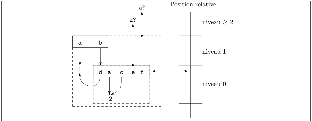
FIG. 6 – Un exemple d'accès à de multiples redéfinitions d'identificateurs. La représentation graphique correspond à l'expression (5). La définition des systèmes peut se représenter sous la forme d'un arbre, où les nœuds correspondent à des systèmes (le premier système défini étant la racine), les sous-systèmes définissent des nœuds et les définitions terminales des feuilles. Les flèches en traits continus indiquent les liaisons, les flèches en traits pointillés représentent les systèmes traversés par les références pendantes, les boîtes en traits ininterrompus représentent des définitions de systèmes, les boîtes en pointillés représentent les inclusions de systèmes.
