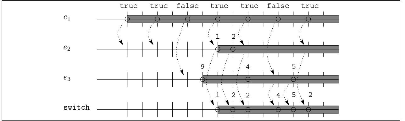
FIG. 4 – Calcul de la valeur de l’expression switch e 1 then e 2 else e 3 . Le domaine de l’expression switch est vrai à partir du moment où les domaines de la condition et de la branche sélectionnée sont vrais. L’expression switch possède un top quand la condition ou la branche sélectionnée possèdent un top. La valeur de switch étant la valeur de la branche sélectionnée par la condition.
