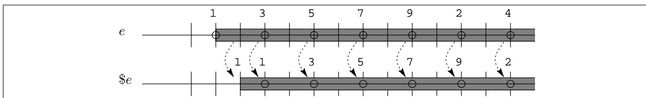
FIG. 1 – Calcul de la valeur de \$e . Les cercles représentent les tops de l'expression ; les barres verticales correspondent aux tics ; les parties grisées représentent le domaine de l'expression.
