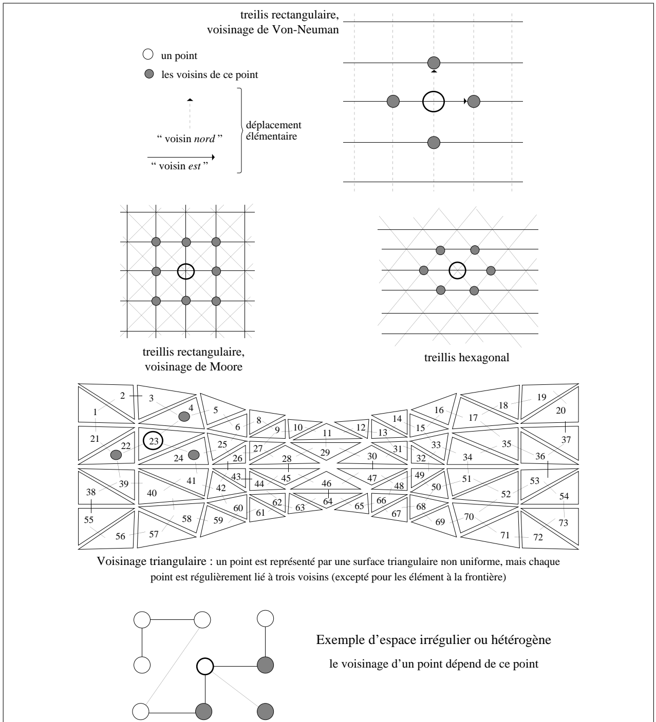
FIG. 1 – Quatre exemples d'espaces homogènes et un exemple d'espace hétérogène.
