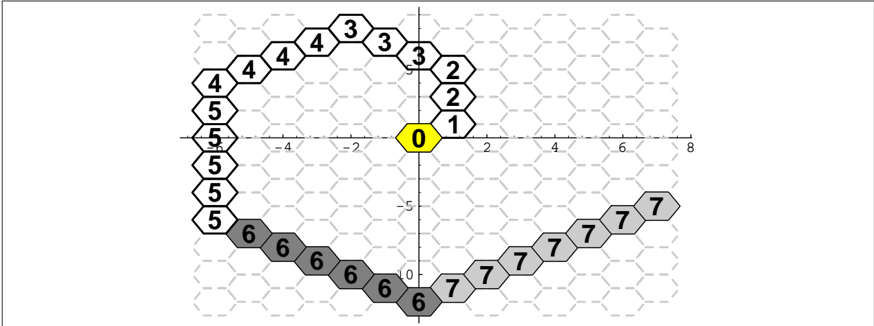
FIG. 7 – La construction d'une spirale sur un réseau hexagonal.
