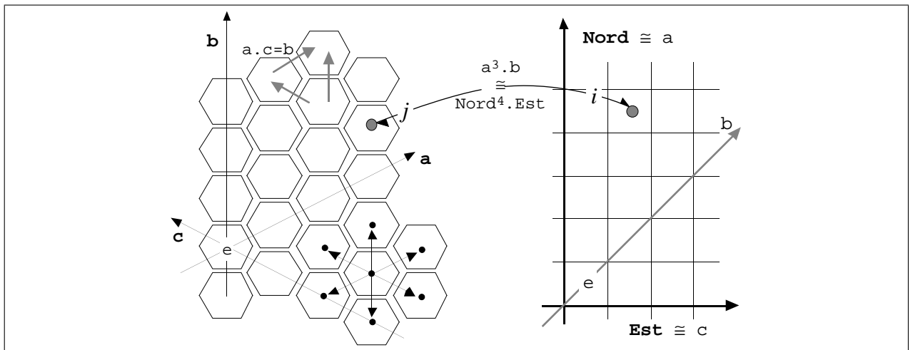
FIG. 4 – Représentation de H^2 et G^2 et de l'isomorphisme entre eux.
