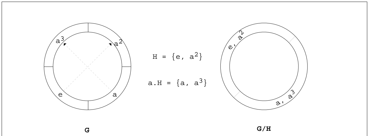
FIG. 10 - Quotient de G = \langle a; a^4 = e \rangle par H = \langle a^2 \rangle : G .
