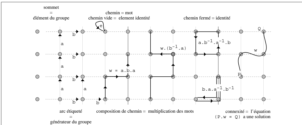
FIG. 3 – Représentation graphique des relations entre les notions de graphe de Cayley et la théorie des graphes.
