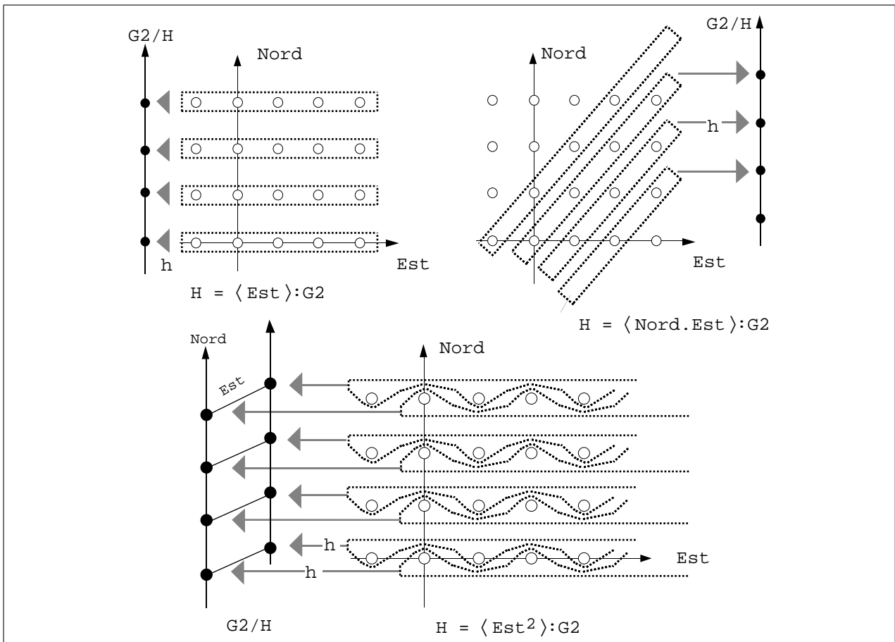
FIG. 14 - Trois exemples de réductions sur la forme G^2 .
