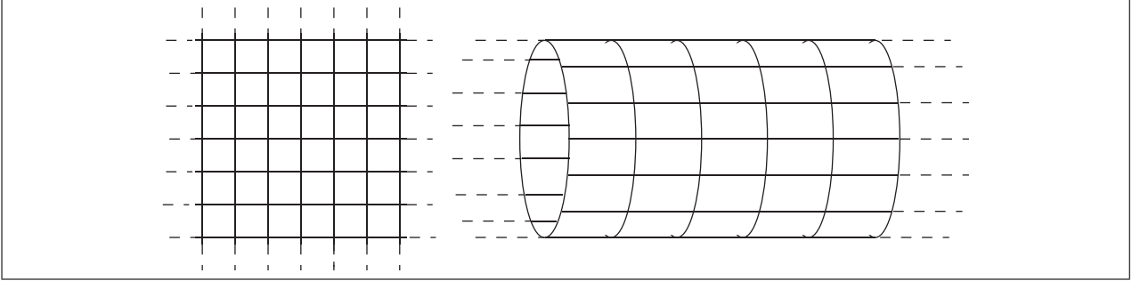
FIG. 1 – Deux exemples de \mathbb{Z} -modules de dimension 2 illustrant le partage entre module libre et module fini. Le premier, \mathbb{Z} \times \mathbb{Z} représente une grille infinie, le second, \mathbb{Z} \times \mathbb{Z}/n\mathbb{Z} , est un tube infini.
