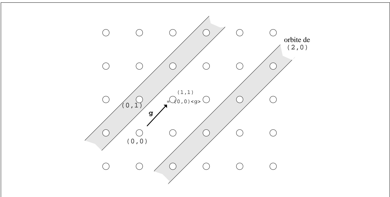
FIG. 2 – Action du groupe G = \langle g \rangle dont les éléments sont les puissances de g , sur l'espace \mathbb{Z}^2 . L'action de g sur \mathbb{Z}^2 consiste à se « déplacer en diagonale ». G n'opère pas transitivement sur \mathbb{Z}^2 : une orbite correspond à une droite diagonale et il y a autant d'orbites que de droites diagonales distinctes.
