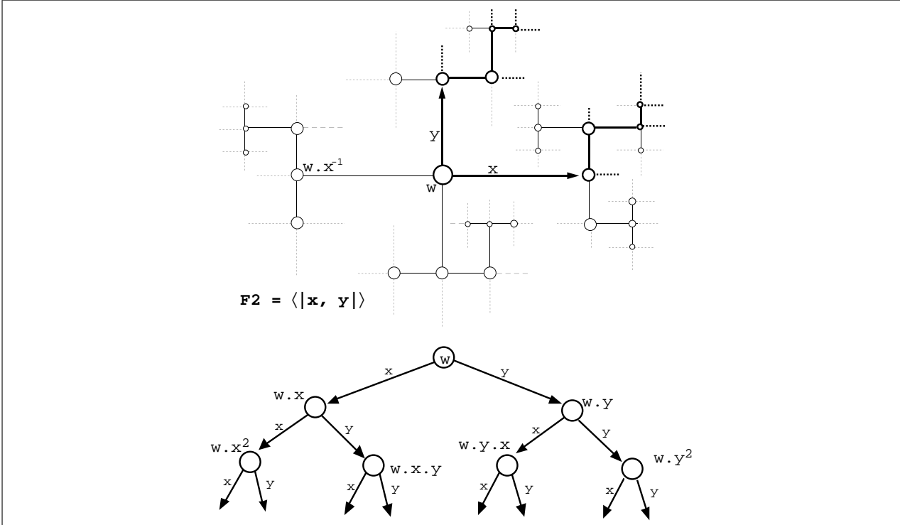
FIG. 7 – Un groupe non-abélien libre avec deux générateurs. Les lignes en gras correspondent à des points qui peuvent être atteints à partir du point w en suivant les déplacements élémentaires x et y .
