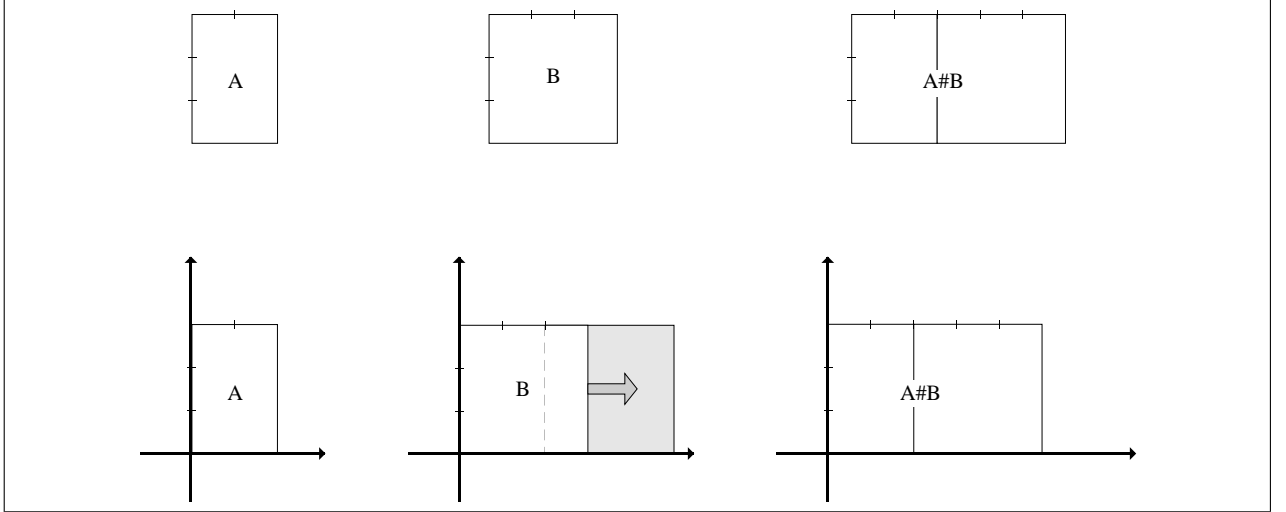
FIG. 13 – Union de deux formes après translation afin d’obtenir un résultat similaire à la concaténation de deux tableaux. La première ligne représente les tableaux à deux dimensions A et B et leur concaténation. La seconde ligne représente ces tableaux comme des régions positionnées dans \mathbb{Z}^2 . La concaténation se traduit par une translation de B de la largeur de A , suivie d’une « union » de régions de \mathbb{Z}^2 .
