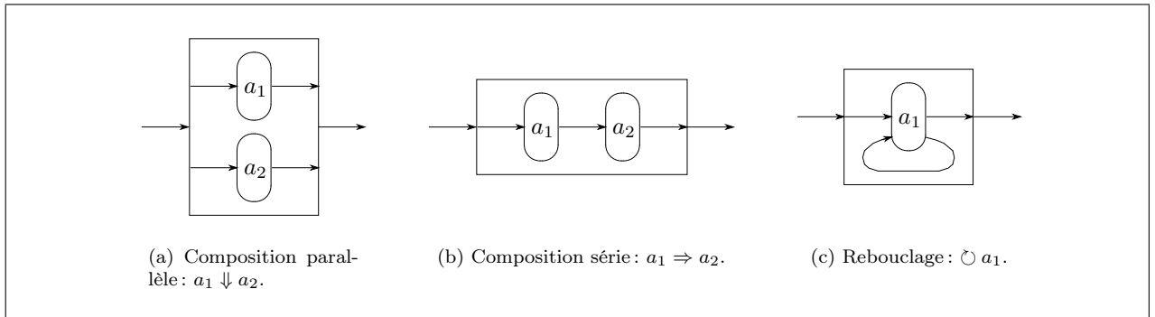
FIG. 5 – Les opérateurs de composition fonctionnelles de DFG : la mise en parallèle, la mise en série et le rebouclage.
