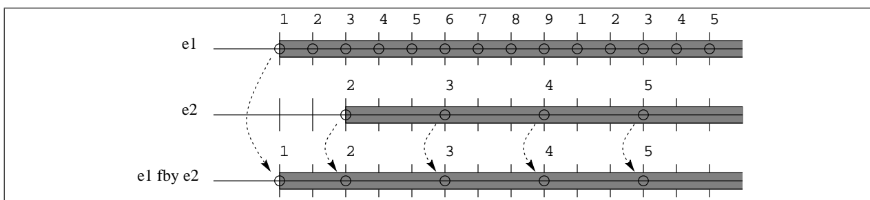
FIG. 2 – Calcul de l'horloge de e_1 \text{ fby } e_2 . L'expression e_1 possède un top tous les tic à partir du premier tic et l'expression e_2 possède un top tous les trois tics à partir du 3 e tic. L'horloge de l'expression fby est celle de e_1 jusqu'au premier top de e_1 puis est égale à celle de e_2 .
