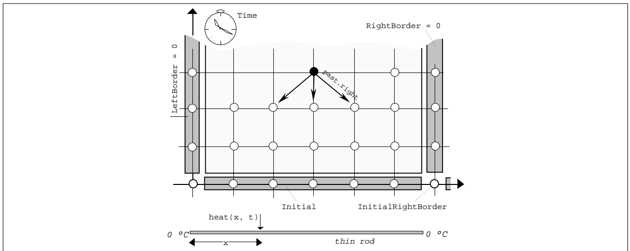
FIG. 2 – Résolution numérique explicite de l'équation différentielle partielle parabolique gouvernant la diffusion de la chaleur dans une barre de métal fine et uniforme.
