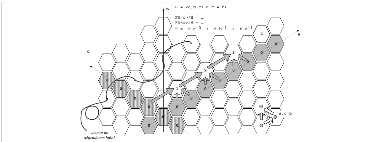
FIG. 17 – Cette figure illustre un champ basé sur une grille hexagonale H = \langle a, b, c; b = a.c \rangle . Le champ F est défini par une expression récursive. Les cosets \langle a \rangle : H et \langle c \rangle : H correspondent aux cas terminaux. L'ensemble de dépendances est \mathcal{DF} = \{a^{-2}, b^{-1}, c^{-1}\} . L'entier qui apparaît dans une cellule correspond à l'instant de production de la valeur de la cellule. À l'instant 0, on connaît la valeur des points des cosets. Les grandes flèches correspondent à un mouvement inverse d'un déplacement de \mathcal{DF} : ces translations peuvent être utilisées pour calculer de nouveaux points à partir des points connus. Dans cet exemple, à chaque instant on ne peut calculer qu'un seul nouveau point. Les cellules qui ont une valeur différentes de \perp ont une frontière plus épaisse. La courbe infinie qui part d'une cellule en maigre montre le début d'un des chemins infinis de dépendances : ce chemin de dépendances « saute » par dessus le coset et part à l'infini.
