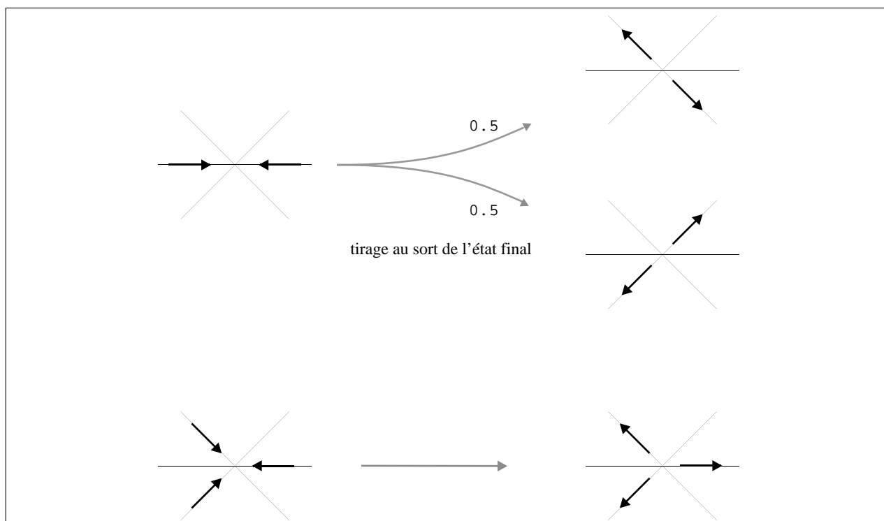
FIG. 4 – Un exemple de famille de règles pour une simulation de gaz sur un réseau à maille hexagonale. Les règles sont représentées aux symétries de rotation près et correspondent au modèle FHP.1 [FHP86]. La règle non-déterministe pour les collisions de type 2 (2 particules en jeu) évite de biaiser le comportement physique malgré la topologie discrète du réseau. Toutes les évolutions de type 1 laissent le vecteur vitesse invariant.
