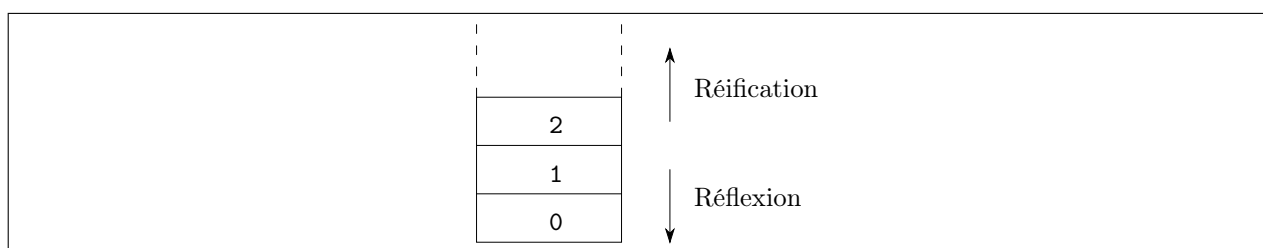
FIG. 1 – La tour d'interprètes dans un langage réflexif
