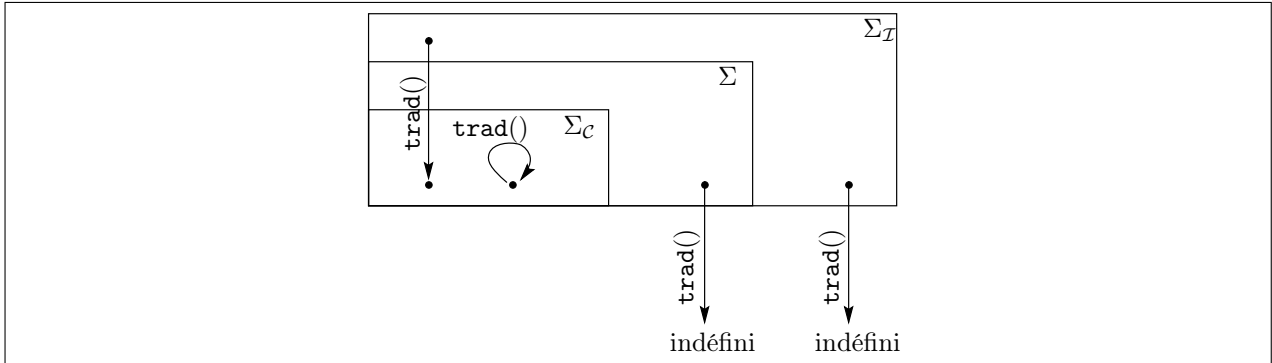
FIG. 2 – La traduction d'un terme de \Sigma_I : si la fonction de traduction est indéfinie, alors la traduction du terme est une erreur, sinon le terme traduit est un élément de \Sigma_C .
