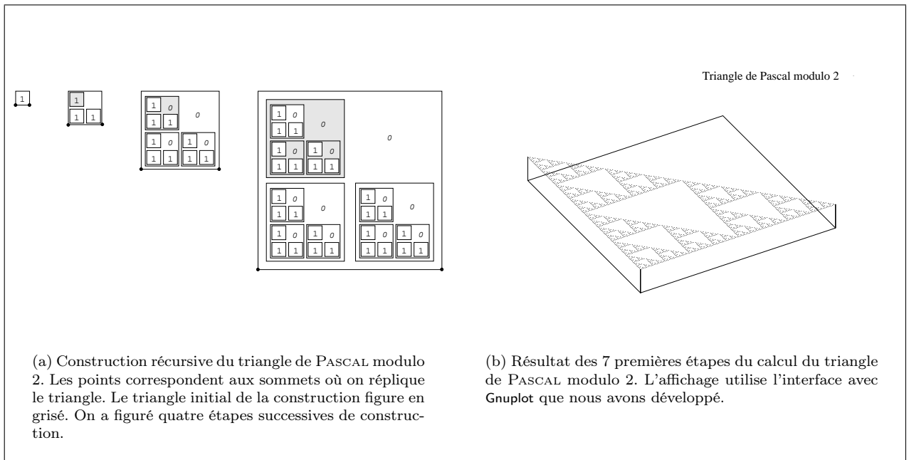
FIG. 2 – Le calcul du triangle de Pascal modulo 2. Détail et résultat de l'exécution du programme 8_{1/2D} .
