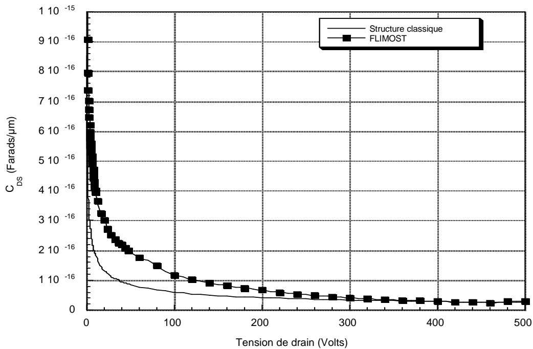
Figure II.24 : Évolution de la capacité C_{ds} en fonction de la tension de drain de la structure FLIMOS à 9 îlots flottants et la structure VDMOS conventionnelle 900 Volts.
