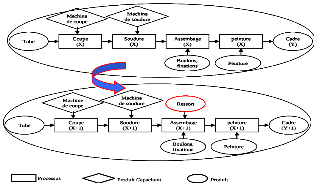
Figure 4.18. processus de fabrication du cadre du vélo.
