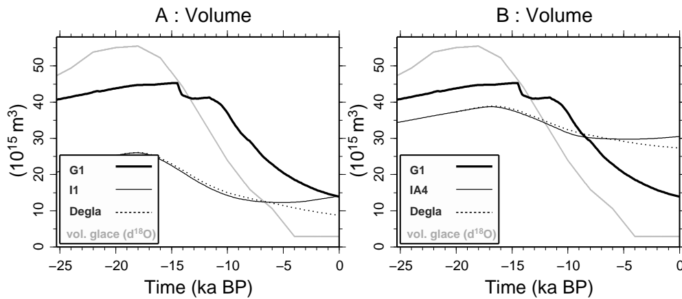
FIG. 7.12: Volume de glace pendant la déglaciation, on compare le niveau des mers, l'expérience G1 basée sur GRIP, et les expériences basées sur l'insolation. Les volume en pointillés (notés Degla) sont obtenue en maintenant l'insolation élevée pendant tout l'holocène. A) expérience I1, et B) expérience IA4, avec albédo.
