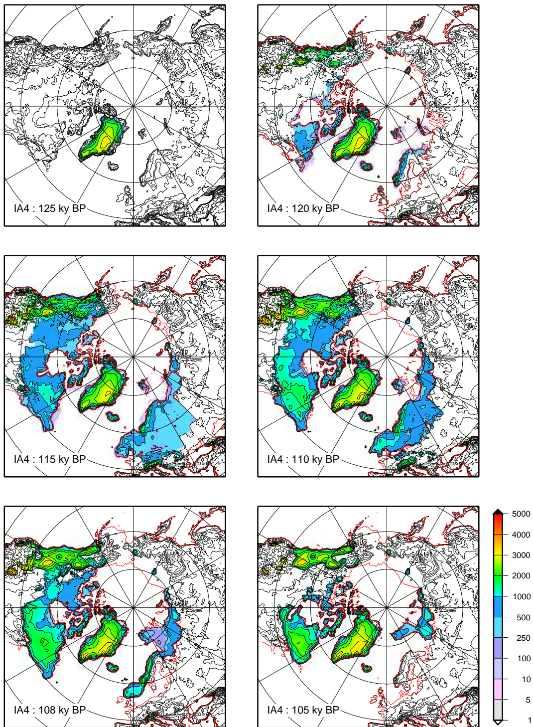
FIG. C.1: Surface des calottes dans l'expérience IA4 entre 125 et 105 ky BP. Le ligne d'échouage est indiquée en rouge.
