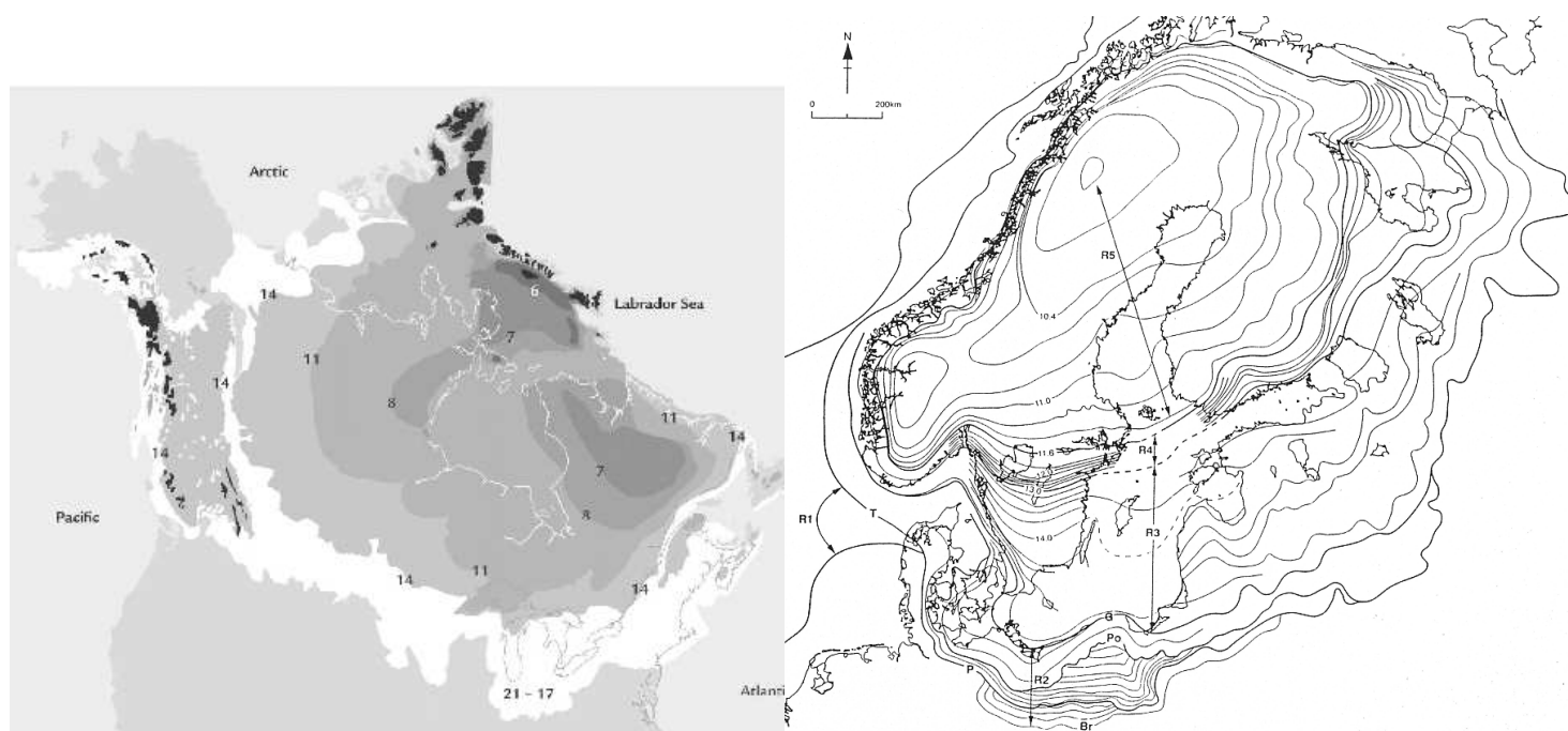
FIG. 5.14: Déglaçiation de la Laurentide (image de Ruddiman et al. (2005)) et de la Fennoscandie (Boulton et al., 2004).
