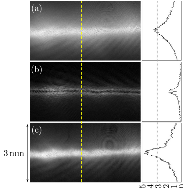
FIGURE 6.12 – Trois mesures de profondeur optique effectuées sur un même nuage atomique comprimé. Sur la droite, on représente le profil de po le long de la ligne tireté sur l'image. La mesure est effectuée de trois manières différentes :
