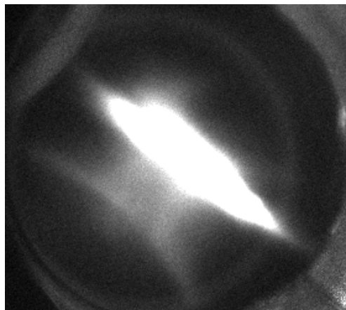
FIGURE 6.4 – Imagerie par fluorescence prise lors du chargement du piège magnéto-optique décrit dans le chapitre 1. Typiquement 10^9 atomes sont éclairés par les 6 faisceaux lasers du piège magnéto-optique dont le désaccord est \delta \approx -3\Gamma .
