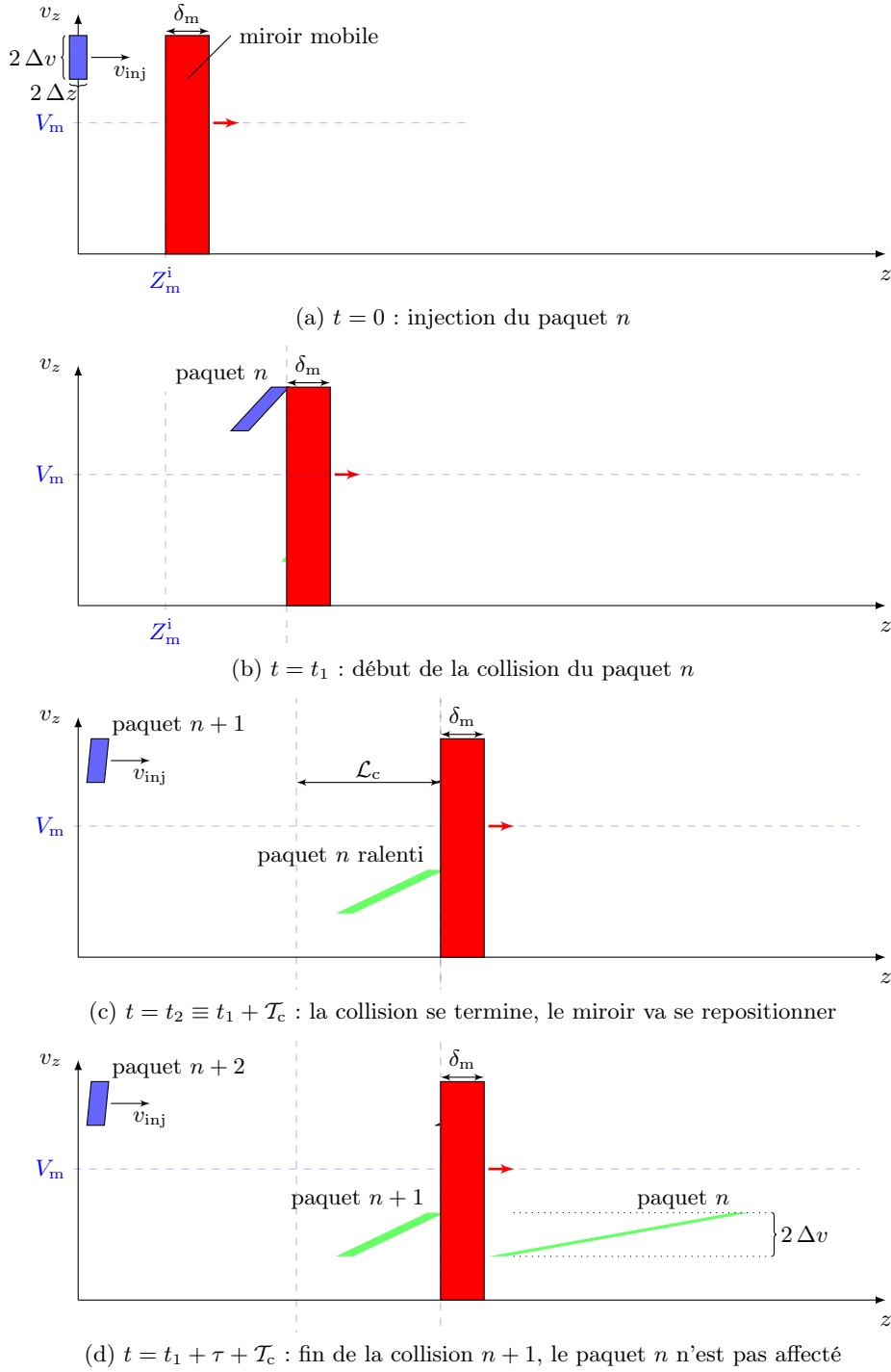
FIGURE 3.11 – Succession de schémas représentant l'évolution des paquets atomiques lors de ralentissements successifs et qui correspondent à : (a) l'instant initial t = 0 d'injection du “paquet n ” ; (b) l'instant t = t_1 du début de la collision avec le miroir mobile ; (c) l'instant t = t_2 \equiv t_1 + \mathcal{T}_c de la fin de la collision ; (d) l'instant t = t_1 + \tau + \mathcal{T}_c de la fin de la collision avec le “paquet n + 1 ”. Il faut alors que tous les atomes du “paquet n ” aient quitté la zone d'action du miroir. On comprend l'importance de disposer d'un agencement permettant au miroir de n'agir que sur une distance donnée.
