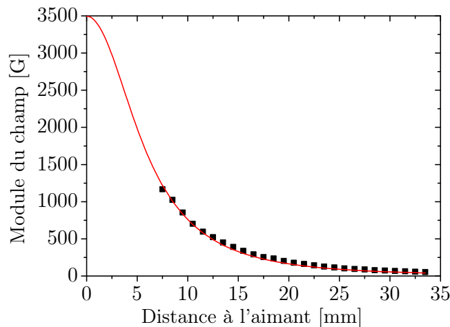
FIGURE E.2 – Mesure de la composante normale du champ magnétique en fonction de la distance à la surface de l'aimant.
