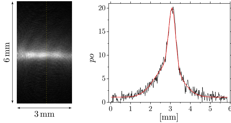
FIGURE 6.11 – Image représentant la profondeur optique po(x, y) = \sigma_0 \rho_c(x, y) d'un nuage atomique dense produit par un piège magnéto-optique bidimensionnel comprimé (du fait de la forme longiligne du nuage, on n'en distingue qu'une partie sur cette image). Le graphe représente le valeur de la profondeur optique le long de la ligne pointillée. Les profondeurs optiques élevées excluent l'utilisation de l'imagerie par absorption faiblement saturante. Afin d'interpréter l'image, nous ajustons une fonction somme de deux gaussiennes qui permet de caractériser la structure bimodale du nuage (la fonction est représentée en rouge sur le graphe).
