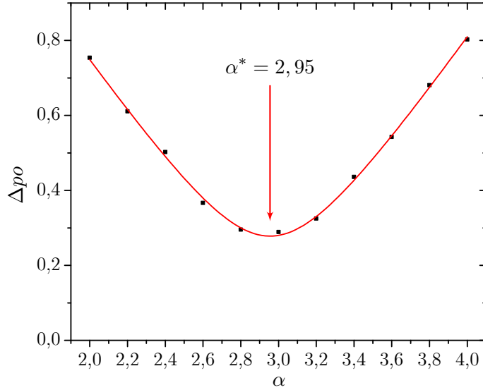
FIGURE 6.10 – Écarts types \Delta po de chaque courbe de la figure 6.9 en fonction de la valeur de \alpha utilisée. La présence d'un minimum pour une valeur \alpha \equiv \alpha^* = 2,95 est déduite par ajustement d'une fonction hyperbolique (ligne rouge).
