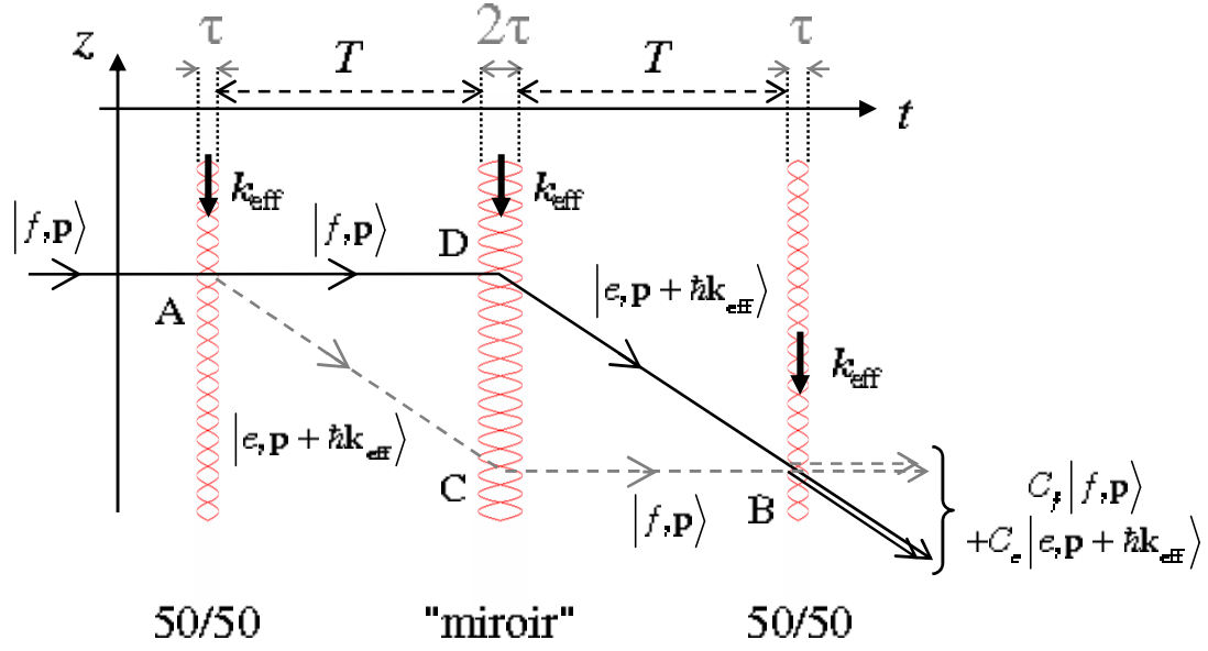
FIG. 2.2 – Schéma d'un interféromètre atomique où les ondes de matières sont séparées puis redirigées et recombinaées par des transitions Raman stimulées. Ces séparatrices lumineuses sont sélectives en vitesse et établissent donc une relation univoque entre les états d'impulsion qui forment l'interféromètre et les états d'énergie interne.
