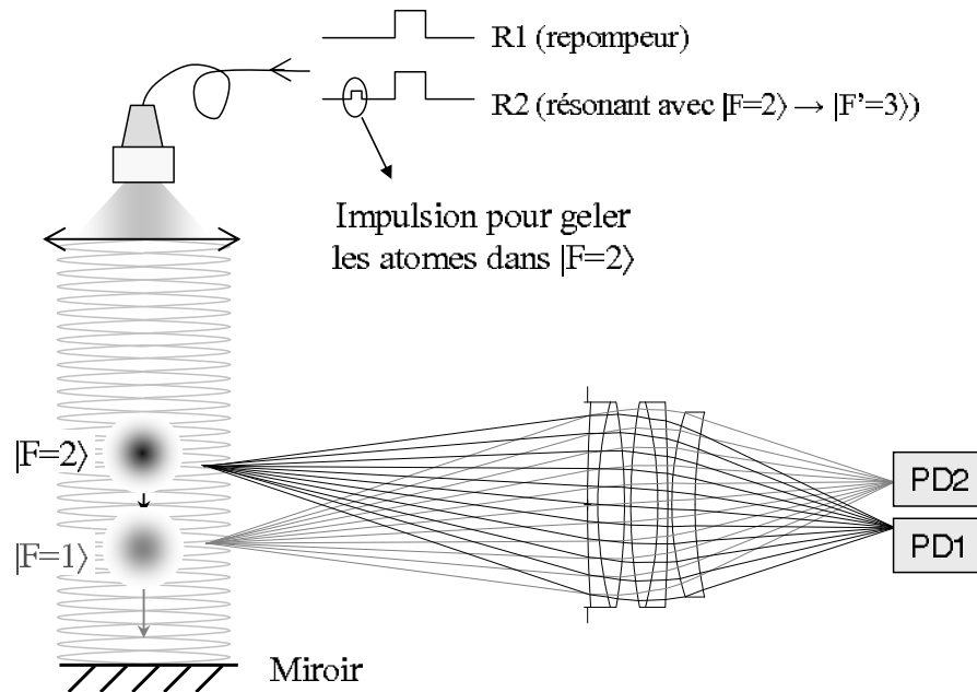
FIG. 3.9 – Schéma de principe de la détection verticale. Les atomes dans |5S_{1/2}, F = 2\rangle sont arrêtés devant la photodiode PD2 par une brève impulsion résonante, tandis que les atomes dans |5S_{1/2}, F = 1\rangle poursuivent leur chute. Une fois devant la deuxième photodiode, une impulsion intense des lasers de repompeur et de détection permet une excitation très efficace des deux populations.
