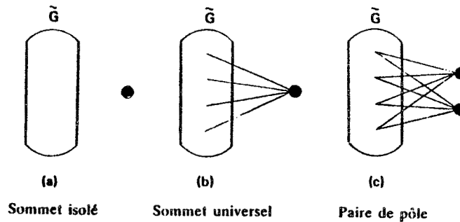
Fig. 1. \tilde{G} est le graphe restant après avoir fait l'une des opérations \phi_1 , \phi_2 ou \phi_3 .
