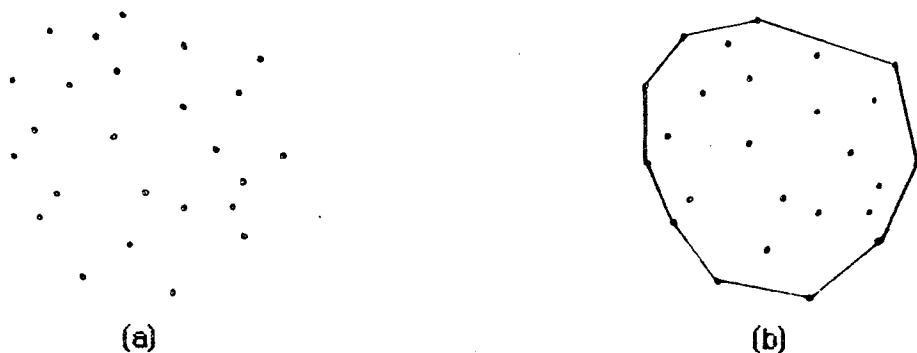
enveloppe convexe des points de la Fig.1 (a)
