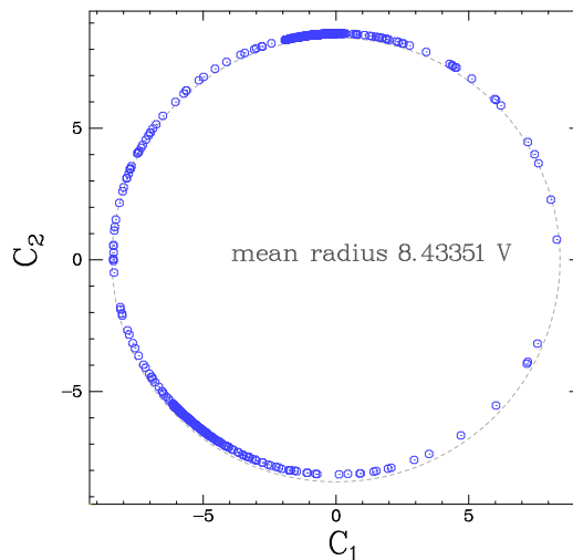
FIG. 2.4 – Visualisation à l'oscilloscope du contraste : C_2 est tracée en fonction de C_1 . Un cercle est alors visible sur l'oscilloscope : les points \circ représentent un échantillon de différentes mesures. La ligne pointillée est la modélisation circulaire des résultats. Le rayon du cercle dépend de la qualité des surfaces rencontrées par le faisceau laser. Ici le rayon typique est d'environ 8 V, le contraste est alors excellent. Un écart au cercle est visible, conséquence inévitable du réglage optique.
