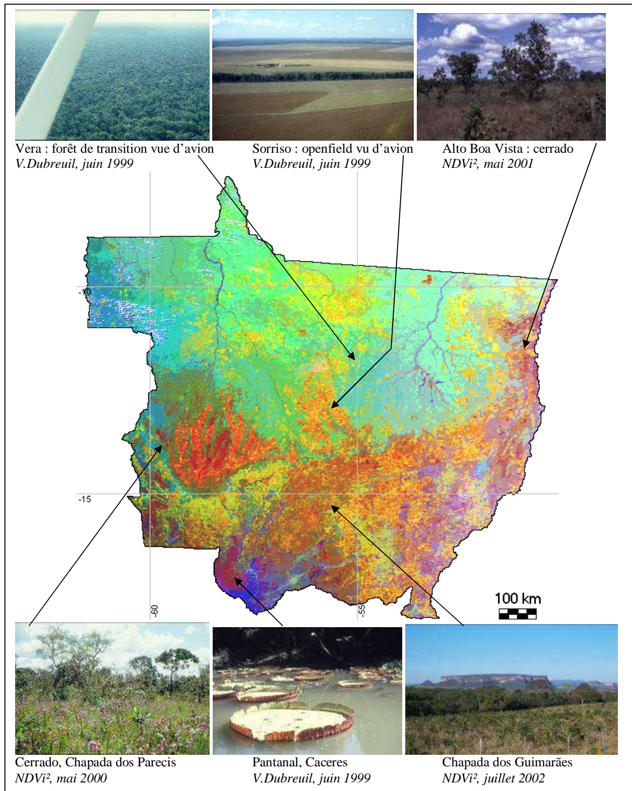
Figure 1.1 : Les grands types de paysages du Mato Grosso : localisation sur une image NOAA-AVHRR du 10/07/1997 (composition colorée 1,2,4) :
