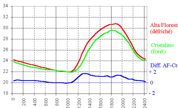
Figure 3.38 : Relevés de température (stations DAVIS-WM2) du 03/04/2003 au 30/04/2003 dans la région d’Alta Floresta : relevés horaires (au dessus) et moyennes sur la période (ci contre). [heure UTC=locale+4]
