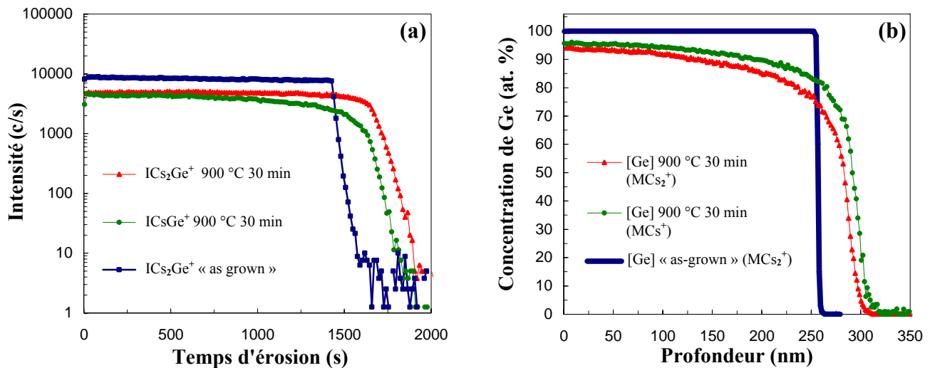
Figure 2.17 : Profils d'intensités secondaires et de concentration respectivement fonction de la durée d'analyse et de la profondeur d'une source solide Ge/Si analysée par SIMS avant et après recuit de diffusion. Les profils de concentration du Germanium ont été déterminés en suivant les méthodologies \text{MCs}_2^+ (b, courbe et motif rouge) et \text{MCs}^+ (b, courbe et motifs vert) appliquées aux variations d'intensités des ions secondaires polyatomiques.
