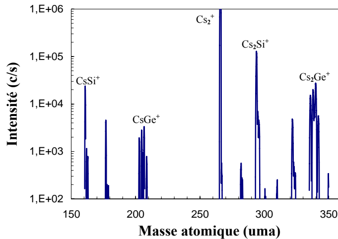
Figure 2.10 : Spectre des masses des ions secondaires positifs d'une hétérostructure \text{Si}_{0,8}\text{Ge}_{0,2} soumise à un bombardement Césium à 1 keV à 45^\circ d'incidence. Sont représentées toutes les espèces présentes dans la gamme de 150-360 uma. Le ratio \text{ICs}_2\text{Ge}^+/\text{ICsGe}^+ est de l'ordre de 8.
