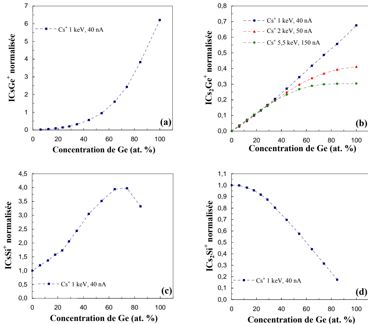
Figure 2.13 : Evolutions des intensités normalisées des ions secondaires polyatomiques associés au Germanium. Les paires CsGe^+ ont été extraites sous bombardement Césium à une énergie d'impact de 1 KeV (angle d'incidence de 45^\circ ) (a). Les clusters Cs_2Ge^+ sont issus de l'analyse Césium à 1 keV (carrés bleus, angle d'incidence de 45^\circ ), 2 keV (triangles rouges, angle d'incidence de 45^\circ ) et 5,5 keV (ronds verts, angle d'incidence de 42,4^\circ ) (b). Les ions secondaires CsSi^+ (c) et Cs_2Si^+ (d) détectés à 1 keV sont également représentés.
