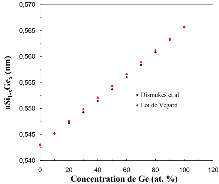
Figure 1.9 : Illustration graphique des écarts des valeurs des paramètres de maille des alliages \text{Si}_{1-x}\text{Ge}_x déterminées par Dismukes et al. et calculées par la loi de Vegard (équation 1.2).
