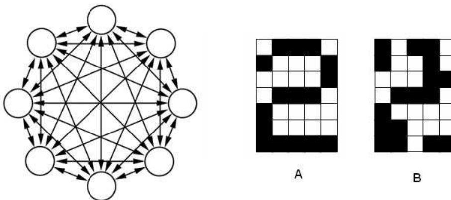
Figure I-23 : Modèle mnémonique de Hopfield (1982) : à gauche, exemple d'un réseau totalement interconnecté, à droite, les deux grilles représentent un état d'un réseau de 35 neurones (image 5x7) : la grille A est le prototype, l'état stable ; la grille B est un état initial (image du '2' bruité) qui convergera vers A.
