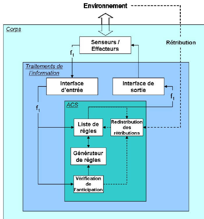
Figure III-16 : Schéma d'un système de classeurs de type ACS
