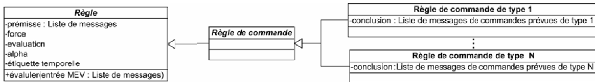
Figure III-21 : Schéma UML simplifié d'une hiérarchie minimale de l'objet « règle ».
