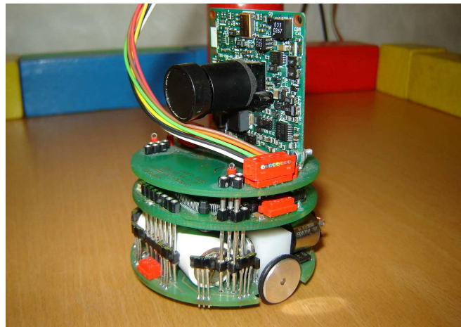
Figure IV-1 : Le robot Khepera.
