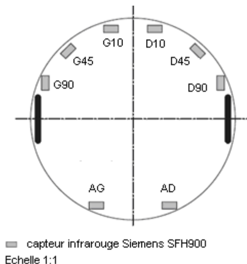
Figure IV-2 : Position des 8 capteurs infrarouges.
