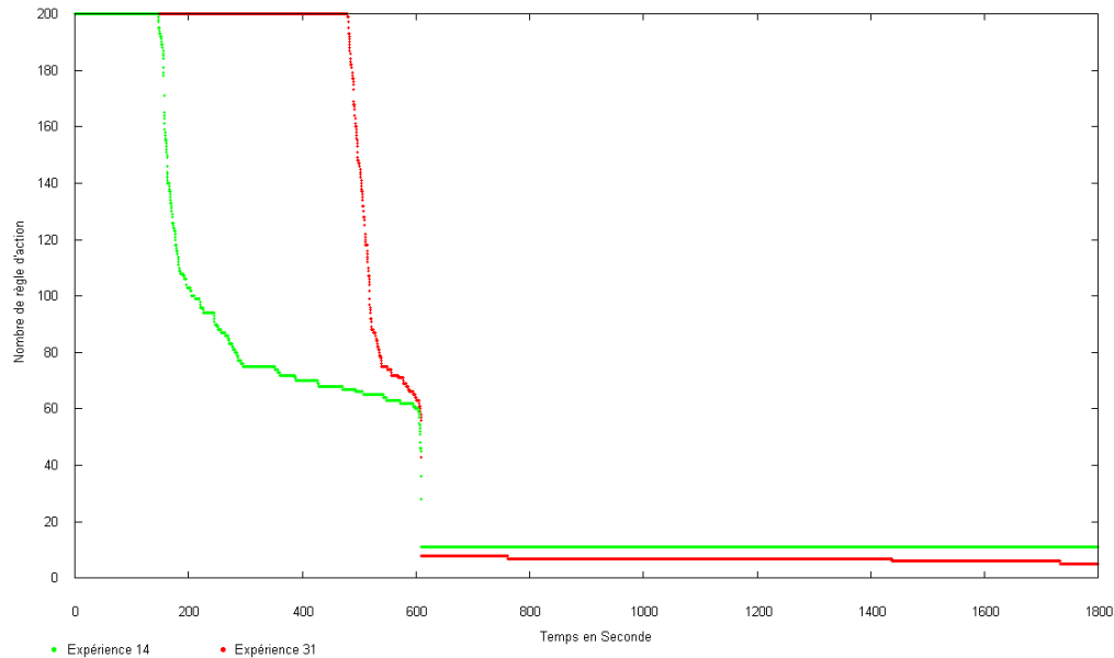
Figure IV-55 : Évolution du nombre de règles d'action dans les expériences 14 et 31.
