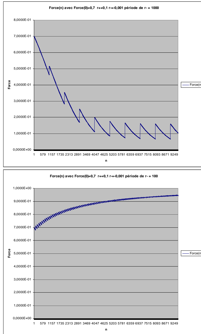
Figure III-32 : Exemple de deux équilibres stables dont la différence de la dynamique provient de la différence entre les fréquences de rétribution positive.
