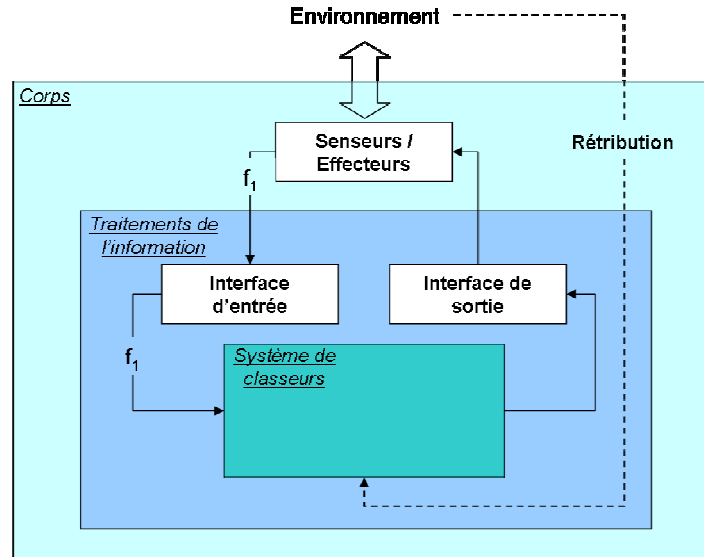
Figure III-12 : Schéma élémentaire d'une architecture de contrôle se fondant sur l'apprentissage par renforcement dans lequel s'inscrivent les systèmes de classeur.
