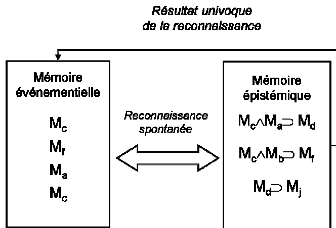
Figure III-11 : Architecture cognitive simplifiée.
