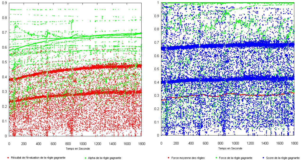
Figure IV-108 : Représentation graphique à droite de l'alpha et du résultat de l'évaluation de la règle déclenchée, à gauche représentation de la force et du score de la règle déclenchée ainsi que la force moyenne des règles de l'expérience 42.
