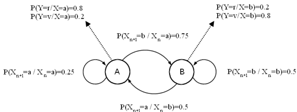
Figure I-33 : Exemple d'un automate markovien avec les variables aléatoires Y correspondant aux observables et X correspondant aux états cachés.
