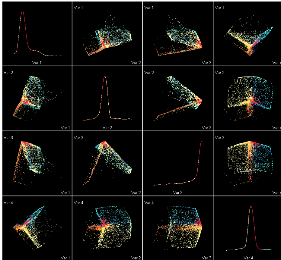
Figure IV-77 : Représentation graphique sensorielle observée au cours de l'expérience 37 : la couleur des points est fonction de la direction de l'effort moteur.
