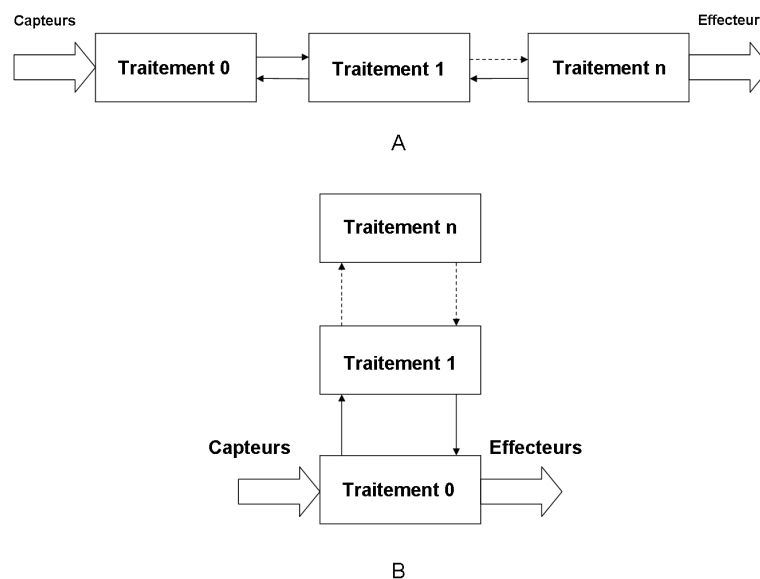
Figure I-31 : Architectures typiques les plus représentatives de l'opposition entre le fonctionnalisme subsymbolique et le fonctionnalisme écologique, respectivement : (A) architecture linéaire et (B) architecture avec subsomption.
