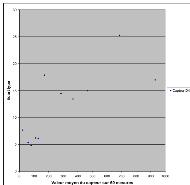
Figure IV-6 : Écart type en fonction de la valeur moyenne du capteur D45.
