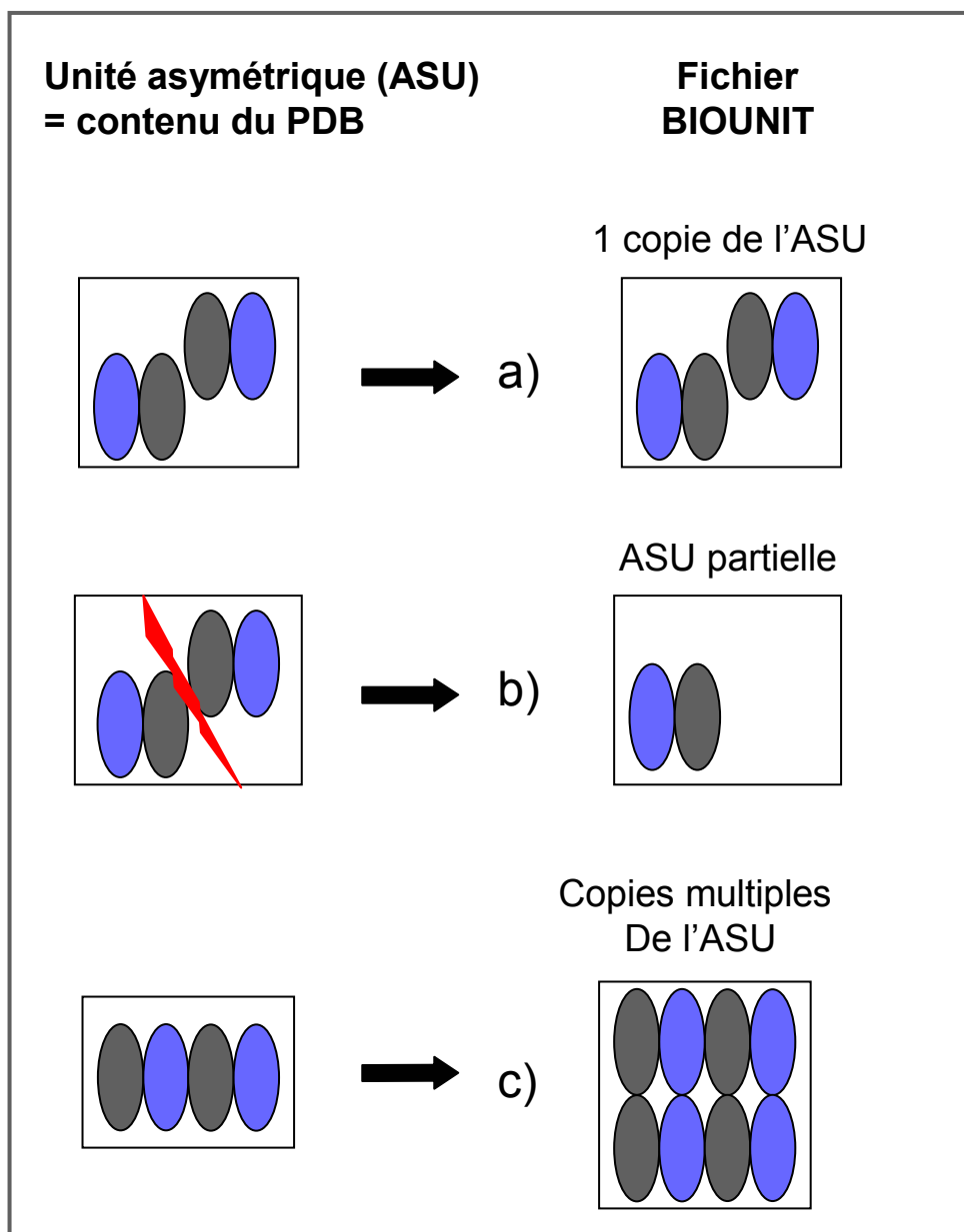
Figure 9. L'unité asymétrique (ASU) est le contenu même du fichier PDB d'origine. Afin d'obtenir le complexe biologique (fichier Biunit), il est parfois nécessaire de dupliquer (c) ou de tronquer le contenu de l'ASU (b).
