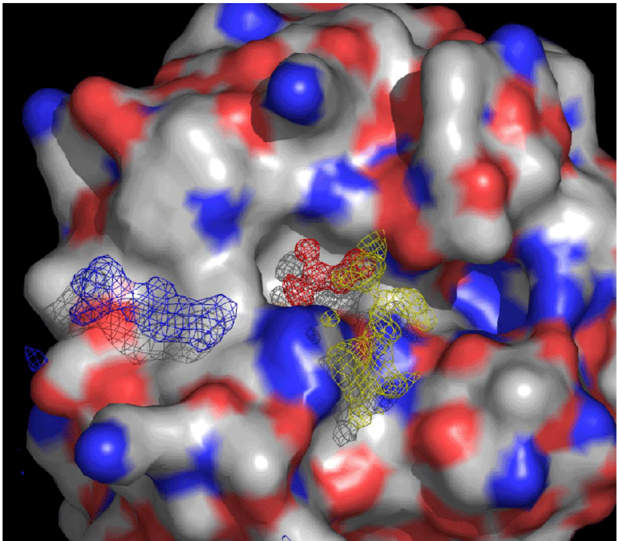
Figure 20 : Superposition de 3 structures cristallographiques de la cyclophiline D centrées sur le site actif et liées à 3 fragments différents représentés par leur densité électronique. La résolution varie de 1 à 1.4 Å.
