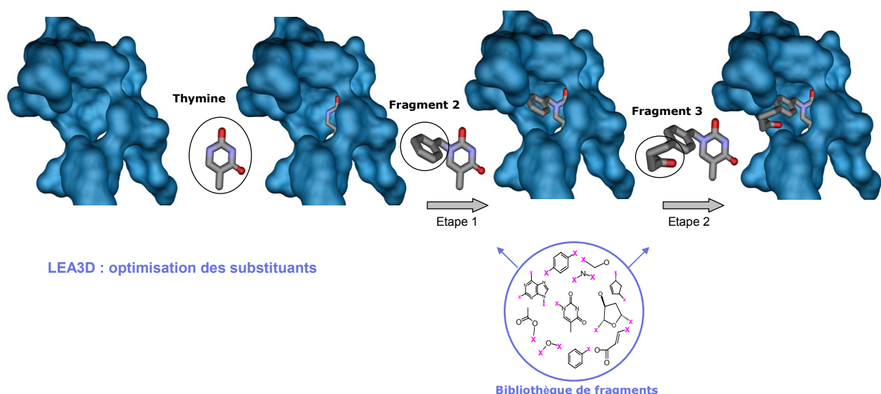
Figure 17 : Optimisation des substituents de la nucléobase thymine par LEA3D en deux étapes.
