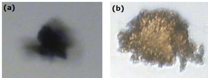
Figure 3.4 – Images optiques d'un grain de la météorite d'Orgueil. (a) Grain avant écrasement ( \sim 30 \times 30 \mu\text{m}^2 ). (b) Grain après écrasement ( \sim 35 \times 49 \mu\text{m}^2 ).
