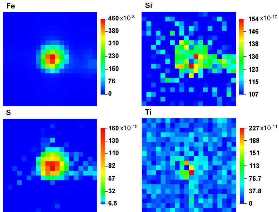
Figure 2.13 – Cartes de la distribution de Fe, Si, S et Ti dans la particule finale de l'échantillon C2009 27mar06. L'échelle de couleur est donnée en nombre de coups (pour un temps de comptage de 2s) normalisé par le nombre de photons incidents. \text{Pixel}=1 \times 1 \mu\text{m}^2 .
