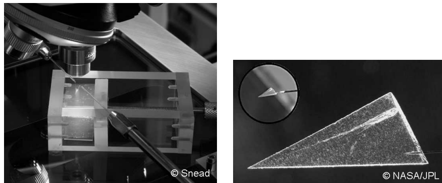
Figure 2.16 – A gauche : Découpe d'un keystone dans un bloc d'aérogel à l'aide de micro-aiguilles au SSL (Berkeley) ; A droite : keystone dans lequel on voit un grain cométaire (au bout de la trace à gauche) et qui a pénétré dans l'aérogel par la droite.
