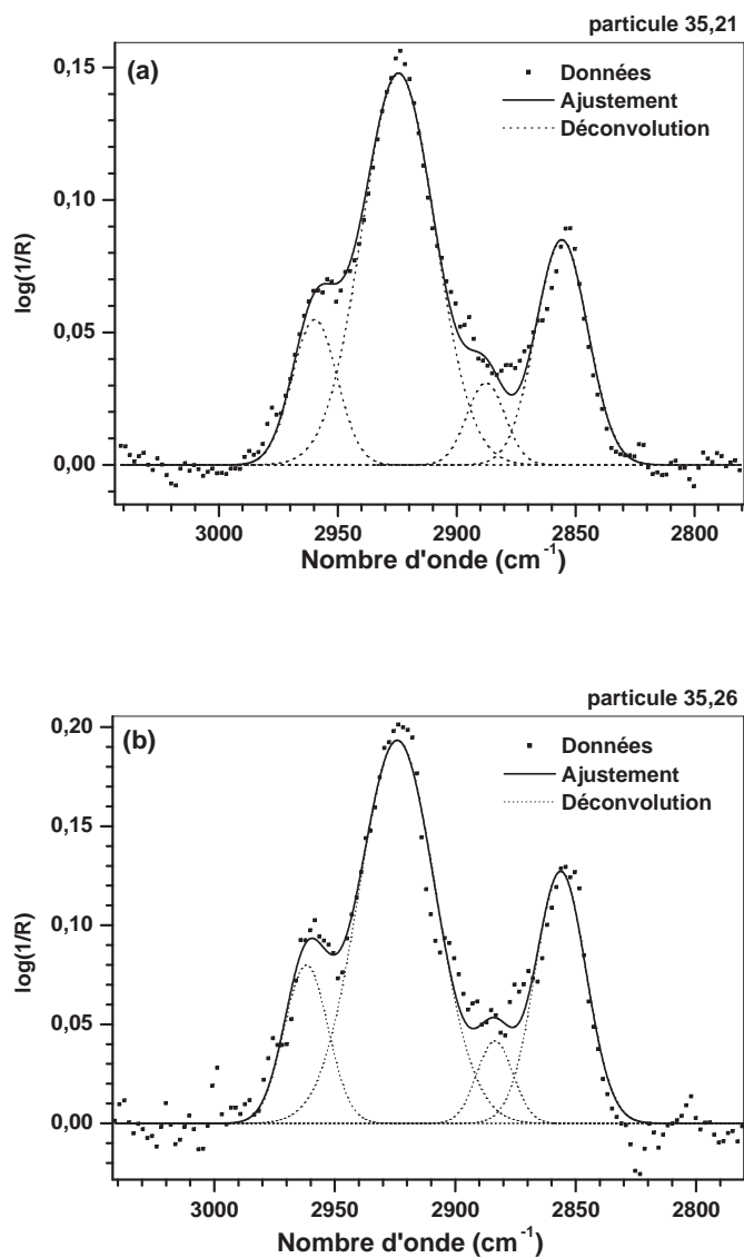
Figure 3.2 – Ajustement à l'aide de quatre gaussiennes de la bande à 3,4\mu\text{m} des échantillons Stardust 35,21 et 35,26.
