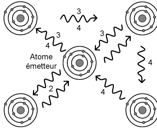
Figure 1.3 – Schéma représentant les phénomènes d'interférence de l'onde associée à l'éjection d'un électron du cœur : (2) diffusion simple (aller-retour), (3) diffusion simple multiple d'ordre 3, (4) diffusion multiple d'ordre 4 (d'après Muñoz (2003)).
