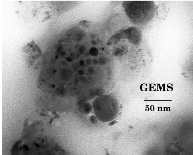
Figure 2.10 – Image MET (champ brillant) d'un GEMS contenu dans un IDP. Les GEMS mesurent généralement quelques 100 nm de diamètre et sont composés de silicates amorphes renfermant des billes d'environ 10 nm, composées de métal et de sulfures à base de Fe et Ni. ©NASA.
