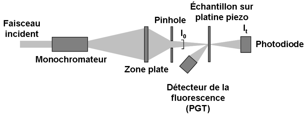
Figure 1.4 – Schéma optique de la ligne ID21 de l'ESRF.
