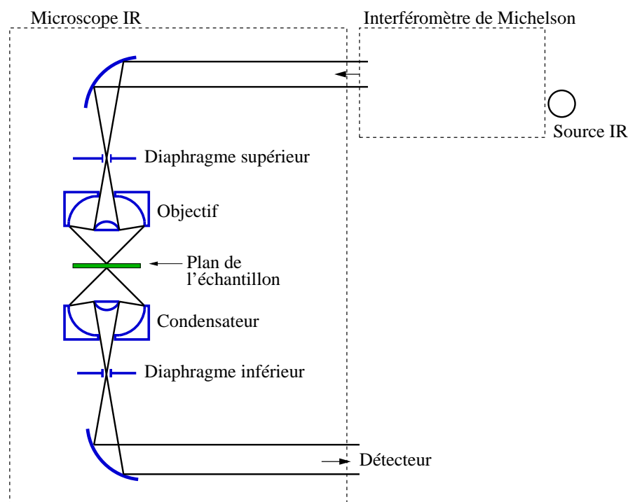
Figure 2.3 – Principe de fonctionnement du microscope IR en mode transmission.
