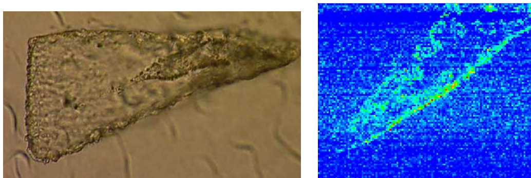
Figure 1.6 – Échantillon LC01B2 (expérience ODCE) : (a) Photo de l'échantillon prise au microscope optique (b) Carte de l'intensité de la bande de fluorescence K_{\alpha} du fer sur laquelle on reconnaît la trace d'entrée.
