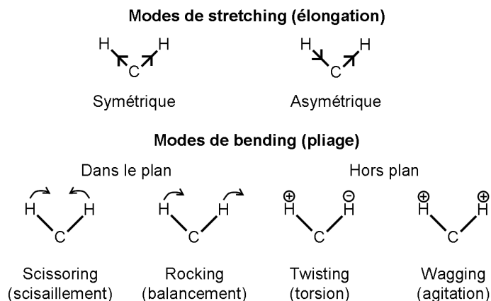
Figure 2.4 – Modes de vibration du groupement méthylène CH_2 .
