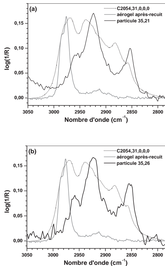
Figure 3.1 – Bande à 3,4\ \mu\text{m} des spectres IR des particules 35,21 (a) et 35,26 (b) comparée à celles du spectre de l'aérogel provenant de la cellule dans laquelle les particules 35,21 et 35,26 ont été prélevées (C2054,31,0,0,0) et du spectre de l'aérogel après recuit. Les spectres ont été normalisés à leur bande la plus intense dans cette région pour mieux visualiser les décalages en nombre d'onde.
