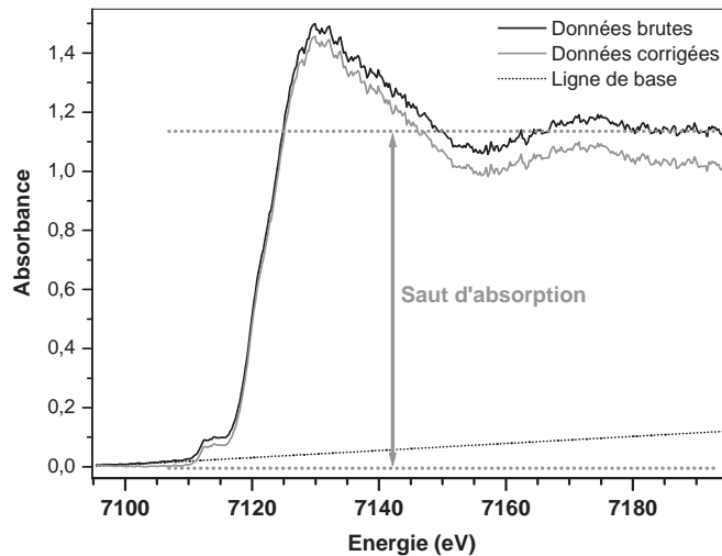
Figure 1.7 – Normalisation d'un spectre XANES.
