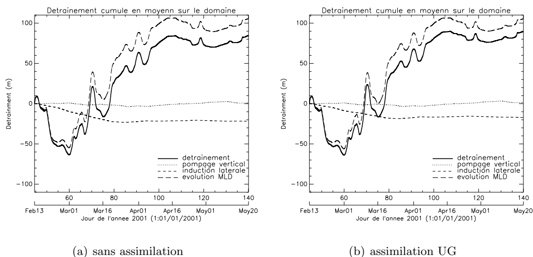
FIGURE 6.16 – Taux de déentraînement intégré dans le temps. Une valeur positive signifie qu'à une date donnée (axe horizontal) la quantité d'eau (en mètre) lue sur l'axe vertical a quitté la couche de mélange depuis le début de l'expérience en moyenne sur le domaine. Les contributions respectives du pompage vertical, de l'induction latérale et de l'évolution temporelle de la profondeur de couche de mélange sont aussi indiquées. L'image de gauche correspond à la simulation sans assimilation, celle de droite à la simulation avec assimilation continue de courant.
