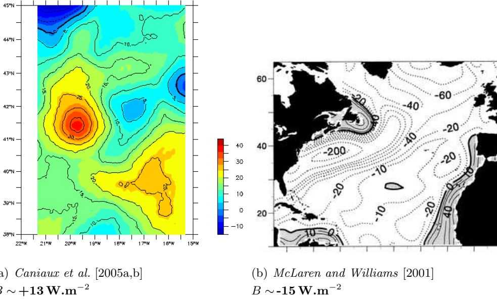
FIGURE 3.1 – Comparaison du flux de flottabilité B exprimé en \text{W.m}^{-2} entre le flux POMME [ Caniaux et al. , 2005a,b] et le flux climatologique de McLaren and Williams [2001]. B = F_{net} - \frac{\beta}{\alpha} \rho_0 C_p \frac{S(E-P)}{1-S/1000} [ Josey , 2003], avec F_{net} le flux thermique net, \beta le coefficient de contraction haline, \alpha le coefficient de dilatation thermique, \rho_0 la densité de référence de l'eau de mer, C_p la capacité calorifique à pression constante de l'eau de mer, S la salinité exprimée en psu, E l'évaporation et P les précipitations. L'expression correcte du flux de sel est en effet \frac{S(E-P)}{1-S/1000} , et non S(E-P) . Cela est lié au fait que la salinité S est exprimée en grammes de sel par kilogramme d'eau salée, et non par kilogramme d'eau douce [ Steinhorn , 1991].
