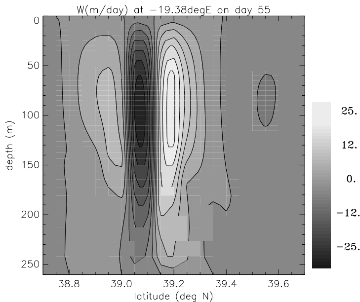
FIGURE 5.12 – Coupe verticale de vitesse verticale (moyenne sur un jour) à 19.38^{\circ}\text{W} le 24 février 2001 dans expMESO. Cette coupe, située juste au sud du tourbillon anticyclonique A2, met en évidence la structure suivant la verticale de deux filaments de vitesse verticale de signe opposé. Les filaments sont situés dans l'océan superficiel, leur largeur est de 10–20 km, et leur intensité atteint plus de 25 m/jour.
