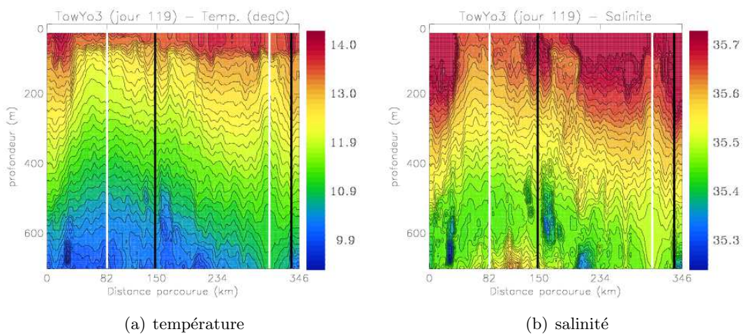
FIGURE 6.10 – Température (image de gauche) et salinité (image de droite) mesurées par le TowYo3 (29 avril 2001, P2L2). Les deux traits blancs matérialisent la position du coeur des tourbillons C5B (kilomètre 82) et A1 (kilomètre 305), respectivement. Les deux traits noirs matérialisent la position de deux bandes d'eau chaude (et salée) dans un environnement plus froid (et moins salé). Figures réalisées par L. Prieur.
