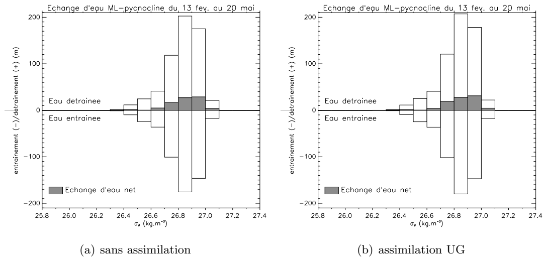
FIGURE 6.17 – Détraînement (barres blanches positives) et entraînement (barres blanches négatives) à travers la base de la couche de mélange (en m) sur des intervalles de 0.1 \sigma_\theta sur le domaine POMME (zone de relaxation exclue). La quantité d’eau nette échangée avec la pycnocline à travers la base de la couche de mélange est représentée par des barres grises. Les champs sont donnés pour toute la durée de la simulation (13 février au 20 mai 2001). L’image de gauche correspond à la simulation sans assimilation, celle de droite à la simulation avec assimilation continue de courant.
