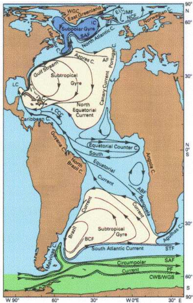
FIGURE 1.2 – Courants de surface dans l’océan Atlantique. Les abréviations sont utilisées pour les courants d’Islande Est (EIC), d’Irminger (IC), du Groenland Ouest (WGC) et des Antilles (AC), et pour le contre-courant des Caraïbes (CCC). Les autres abréviations sont utilisées pour les fronts : front de Jan Mayen (JMF), front du courant de Norvège (NCF), front d’Islande-Féroé (IFF), front subarctique (SAF), front des Açores (AF), front d’Angola-Benguela (ABF), front du courant du Brésil (BCF), front subtropical (STF), front subantartique (SAF), front polaire (PF), limite de l’eau continentale/limite du gyre de Weddell (CWB/WGB). Figure reproduite d’après Tomczak and Godfrey [2001].
