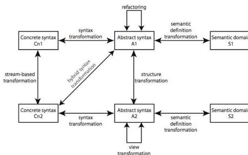
FIGURE 2.11: Classes de transformations dans la définition d'un DSML [Kle06]
