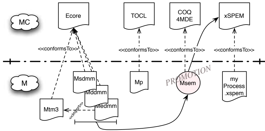
FIGURE 8.8: Description de la promotion dans COQ4MDE
