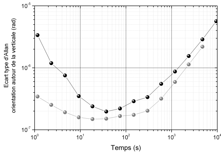
FIG. 5.13 : Ecart-type d'Allan de l'orientation de l'aire interférométrique (points noirs), par rapport à la direction Est-Ouest, mesurée à l'aide de deux capteurs de distance dont les dérives intrinsèques correspondent aux points gris.
