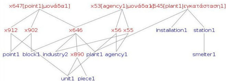
Figure 3. Le semi-treillis décrivant le sens industriel de plant
