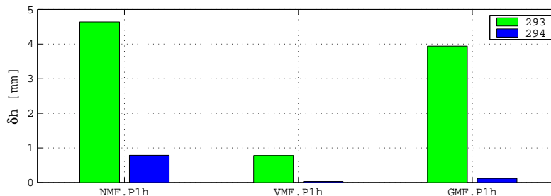
FIG. 3.10 – Écarts entre hauteur estimée et hauteur de référence pour les jours 293 et 294 (20 et 21 octobre 1999) pour des corrections a priori à l'aide des fonctions de projection NMF, VMF et GMF et une mesure de pression sol à 1 h.
